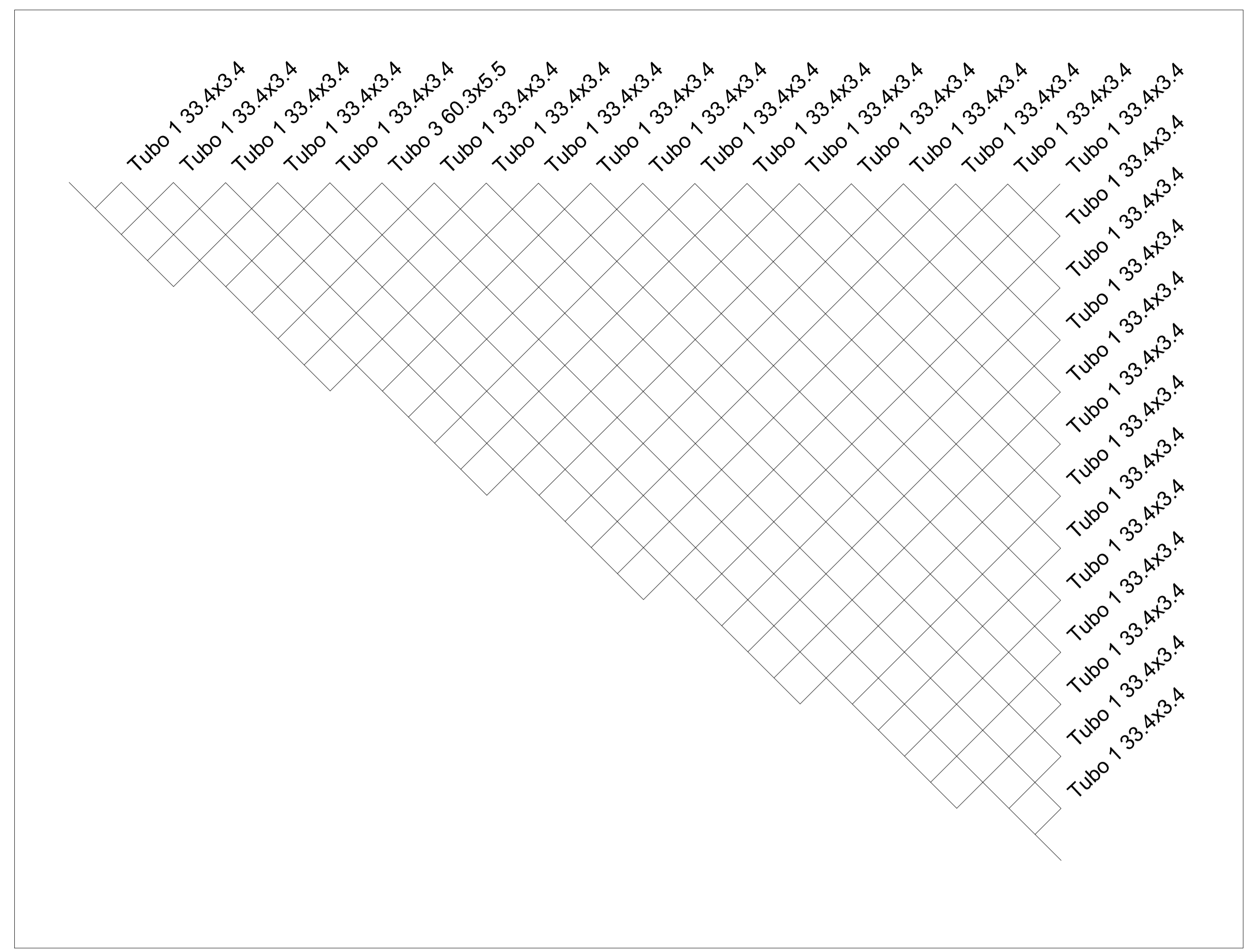
2 MALHA ESPACIAL 02 - DIAGONAL A ESCALA 1:50
