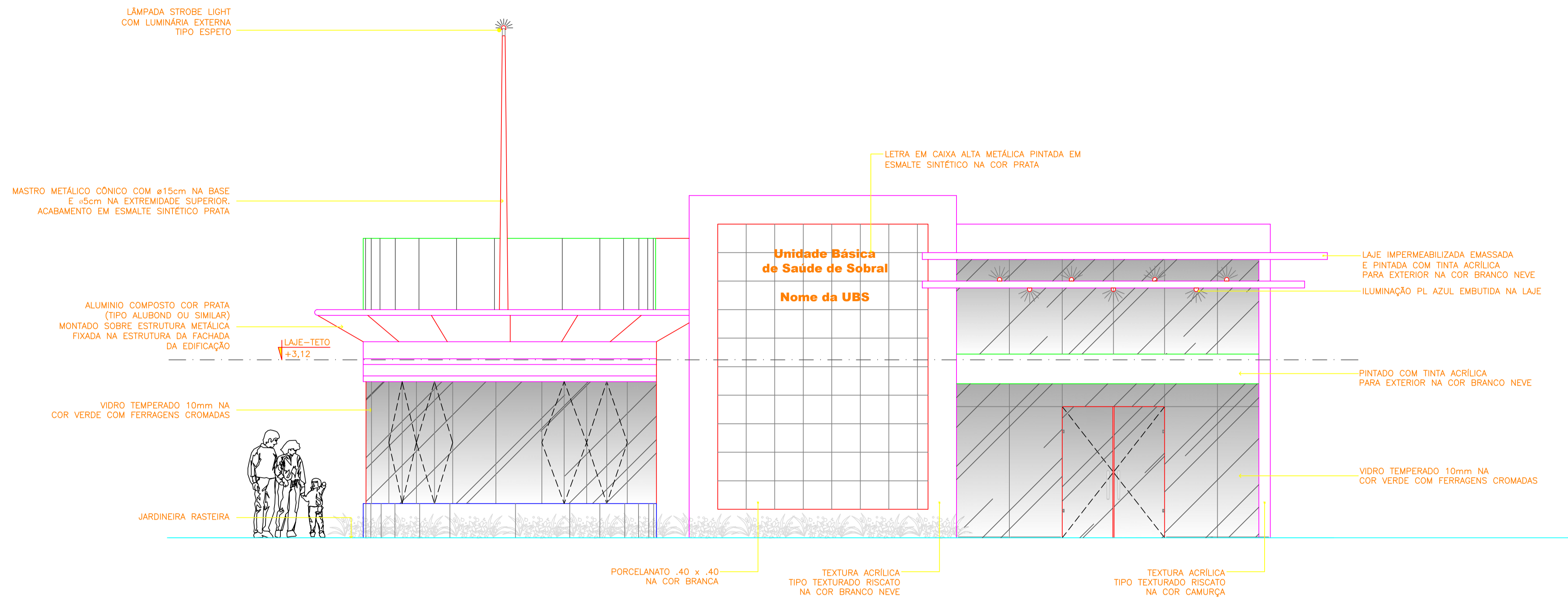
01 FACHADA A- FRONTAL esc: 1/50
