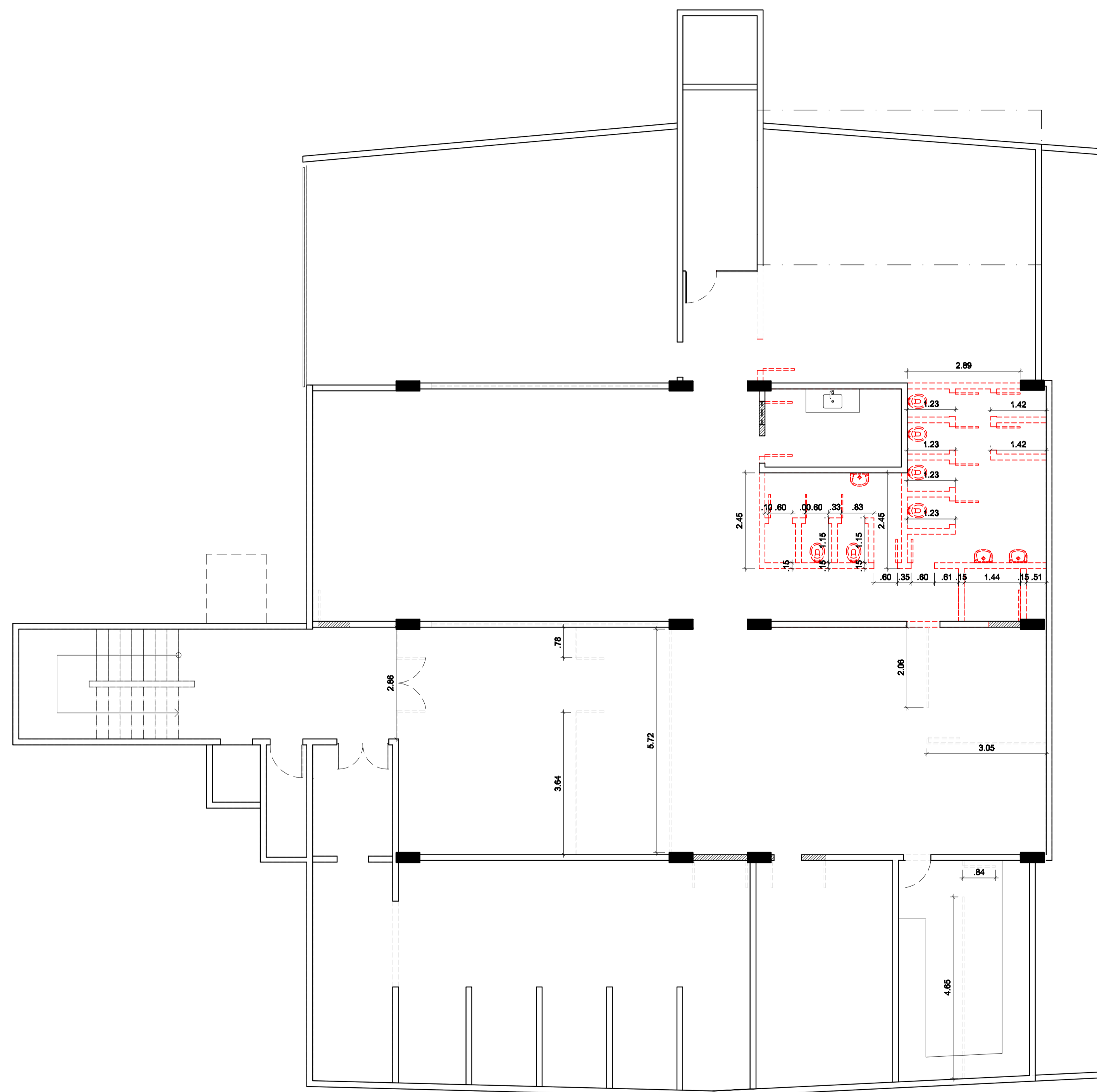
1 PLANTA DE DEMOLIÇÃO SUBSOLO ESCALA 1/75
