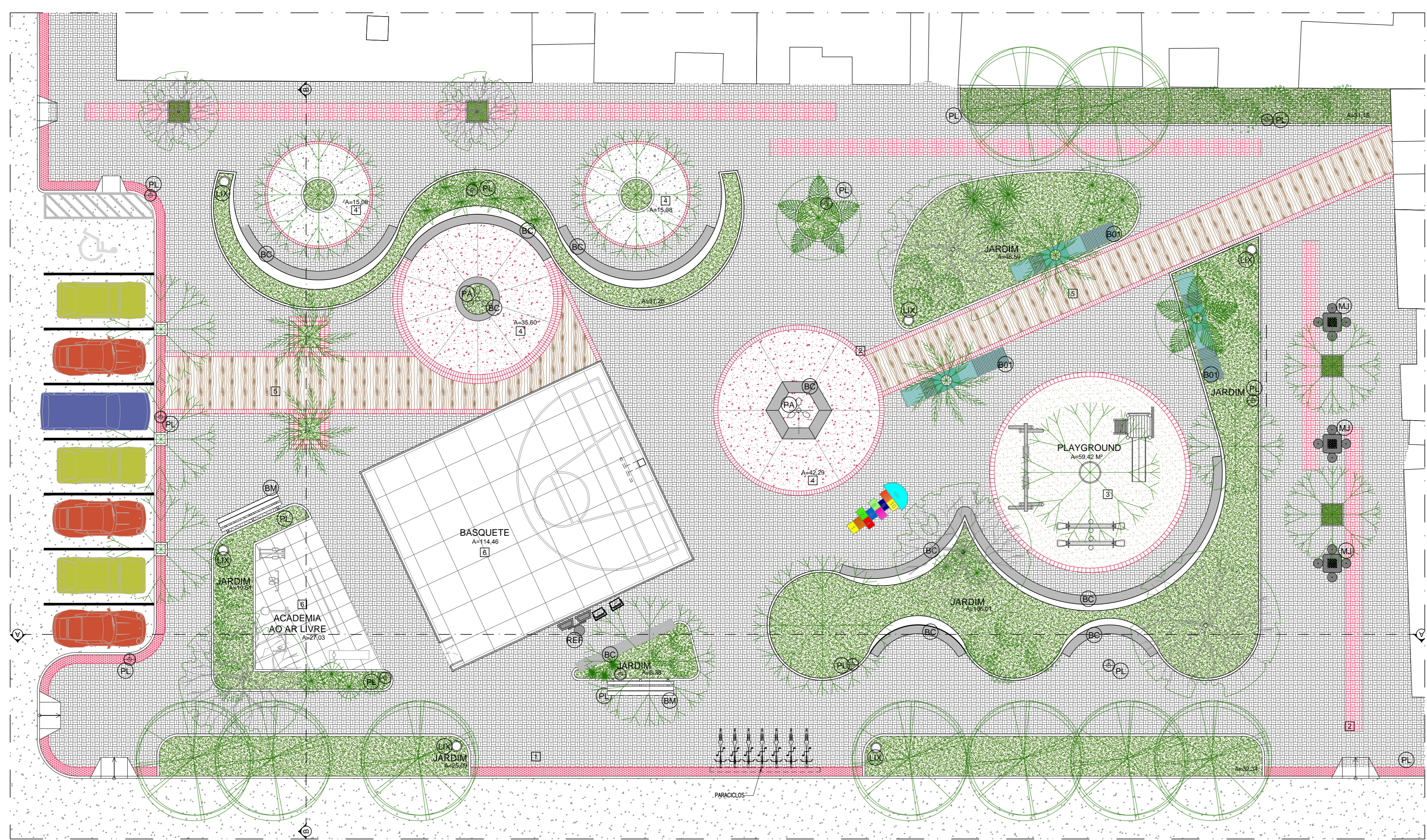
01 PLANTA GERAL
