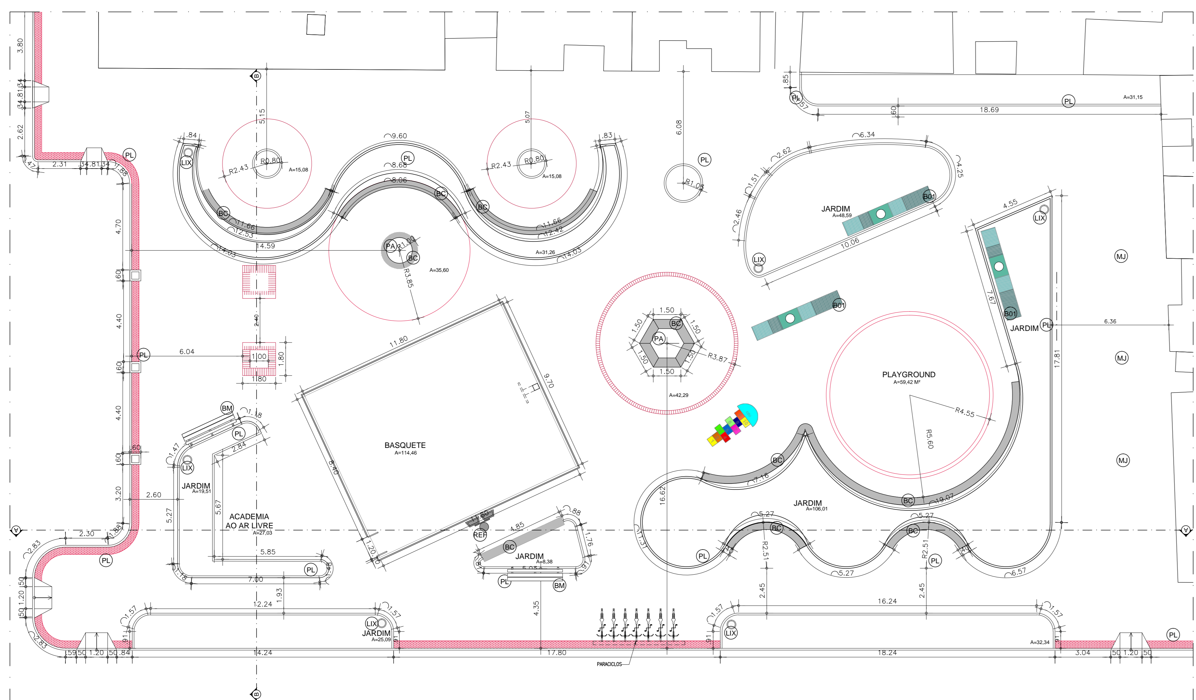
03 PLANTA OBRA
