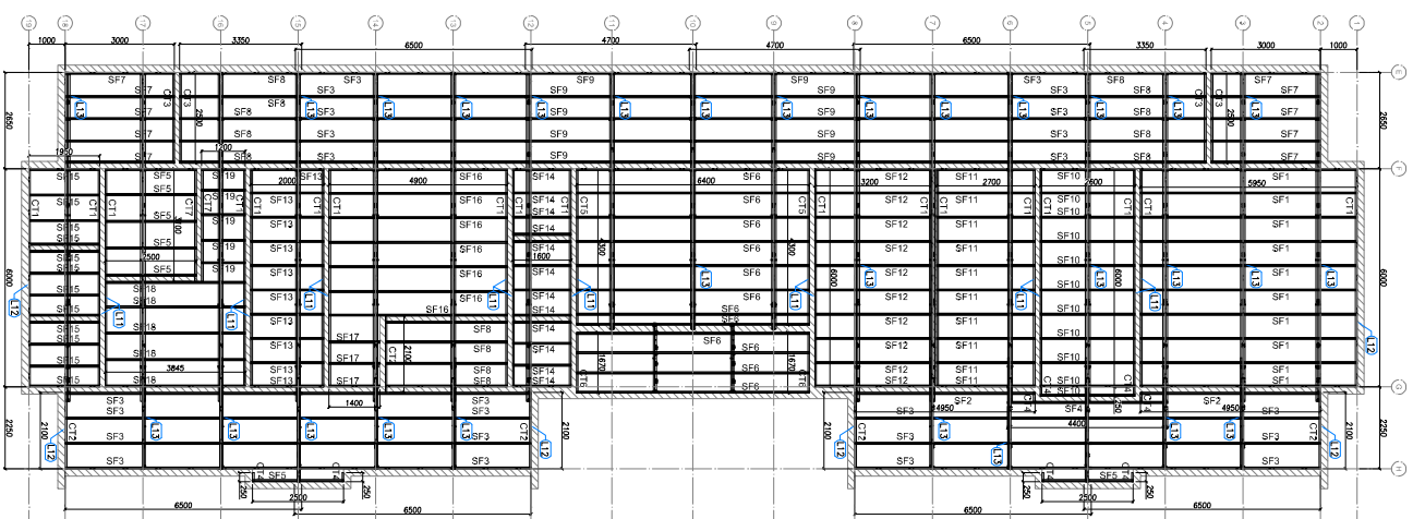
2 BLOCO A - VISTA EM PLANTA APOIOS DO FORRO ESCALA: 1/75
