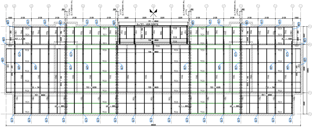
1 BLOCO B - PLANTA DE COBERTURA - CABROS, TESOURAS, TERÇAS, TRAVAMENTOS E LUZAS ESCALA: 1/15
