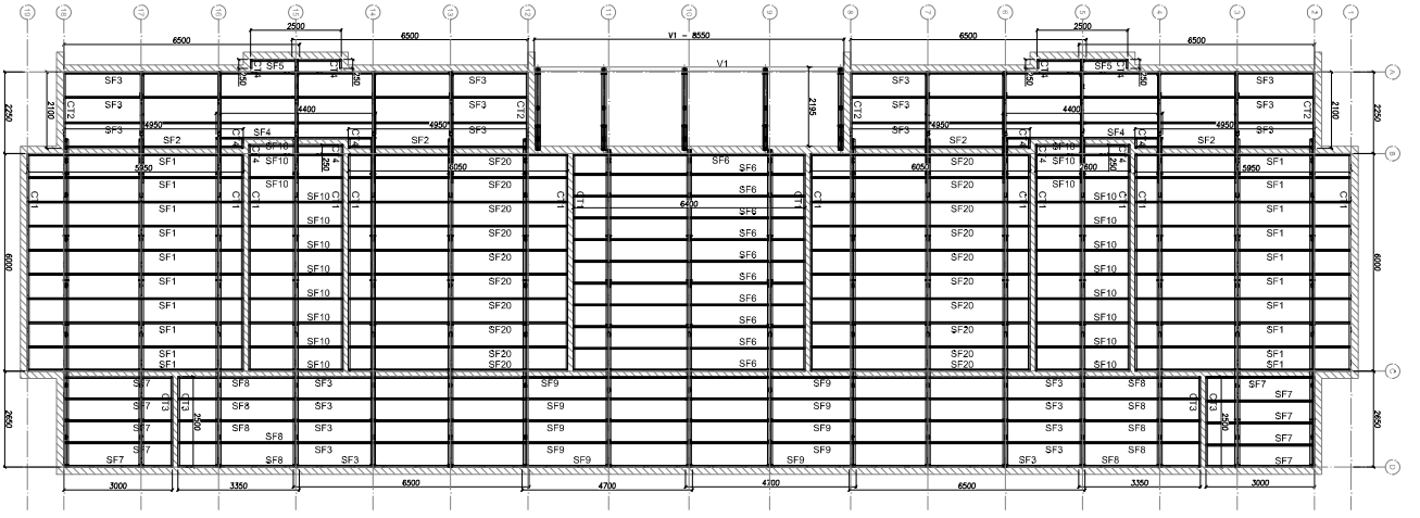
2 BLOCO B - VISTA EM PLANTA SUPORTES DO FORRO ESCALA: 1/15
