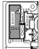
ARMACÃO NEGATIVA DAS LAJES DO PAVIMENTO BALDRAME (EIXO Y)
