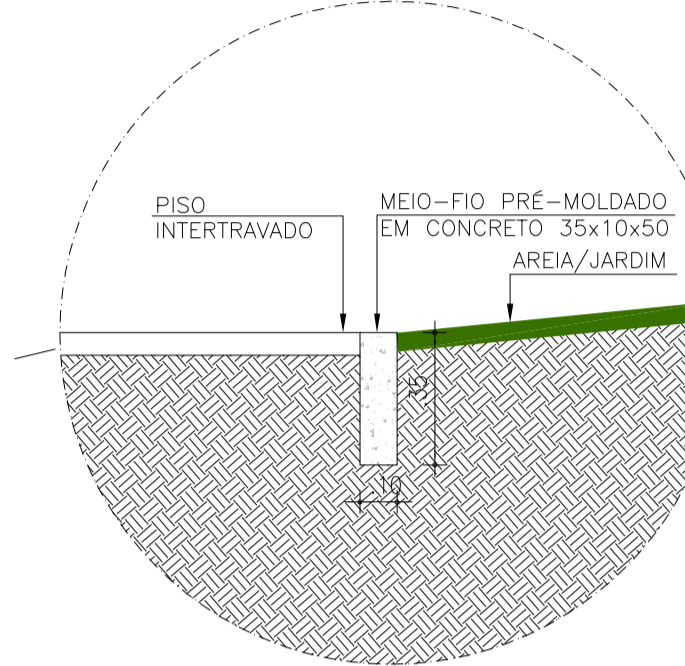
03 DETALHE MEIO-FIO 1/20
