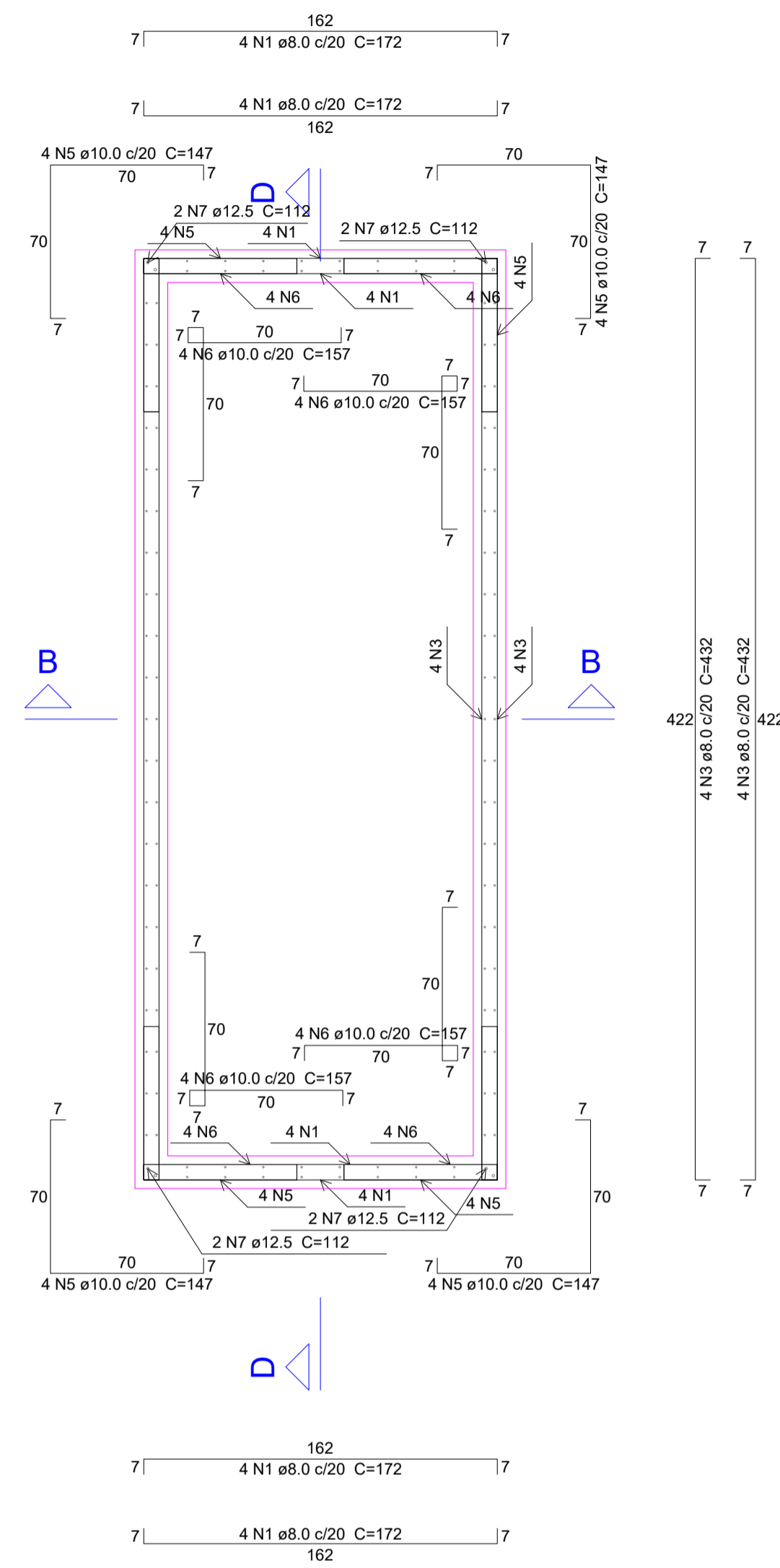
Caixa de Manobra e Tanque de Contato Planta (-33.1) escala 1:25
