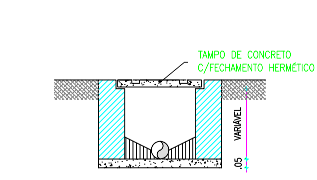
CORTE BB-TAMPA DE INSPEÇÃO ESCALA - 1:20
