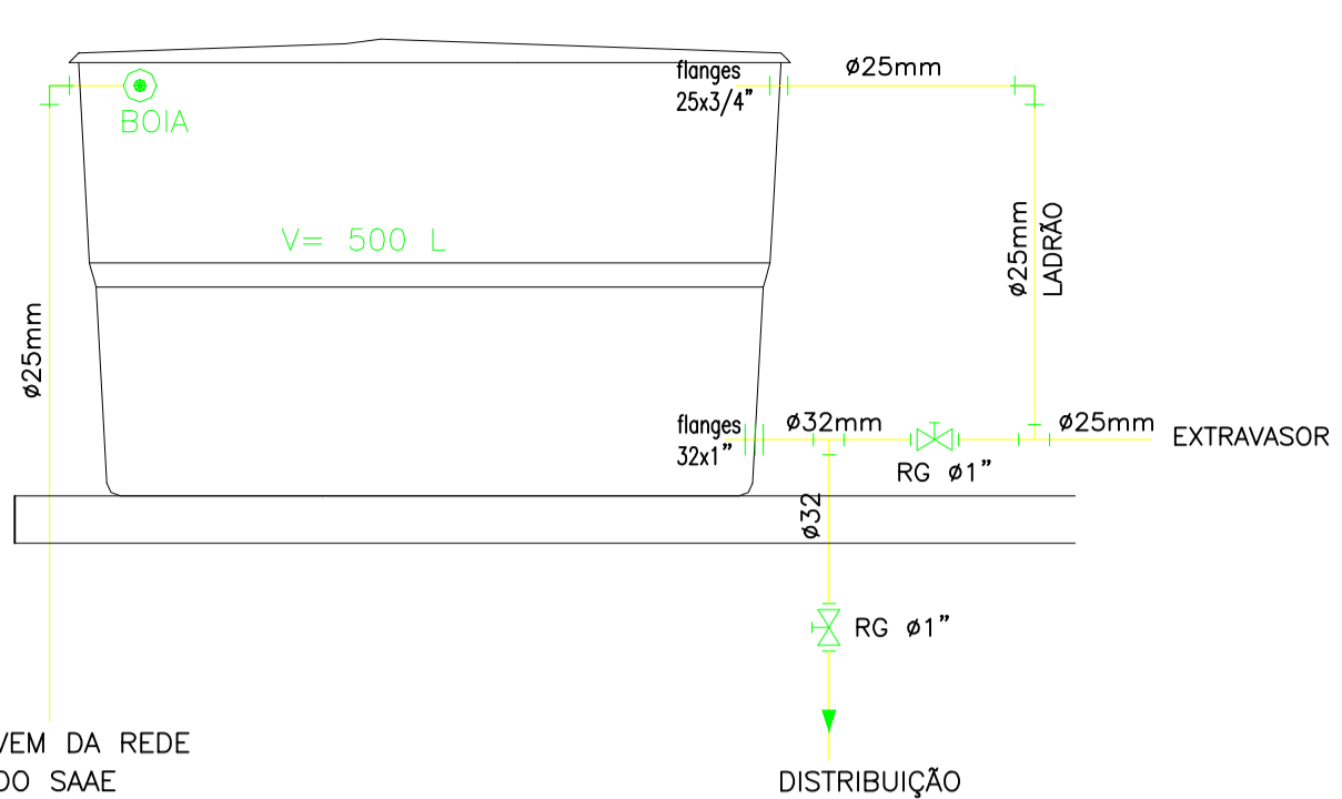
DETALHE CAIXA D'ÁGUA
