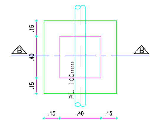
PLANTA BAIXA-CAIXA DE INSPEÇÃO ESCALA - 1:20
