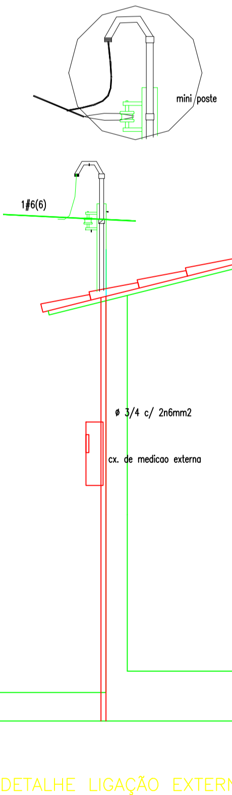
DETALHE LIGAÇÃO EXTERNA
