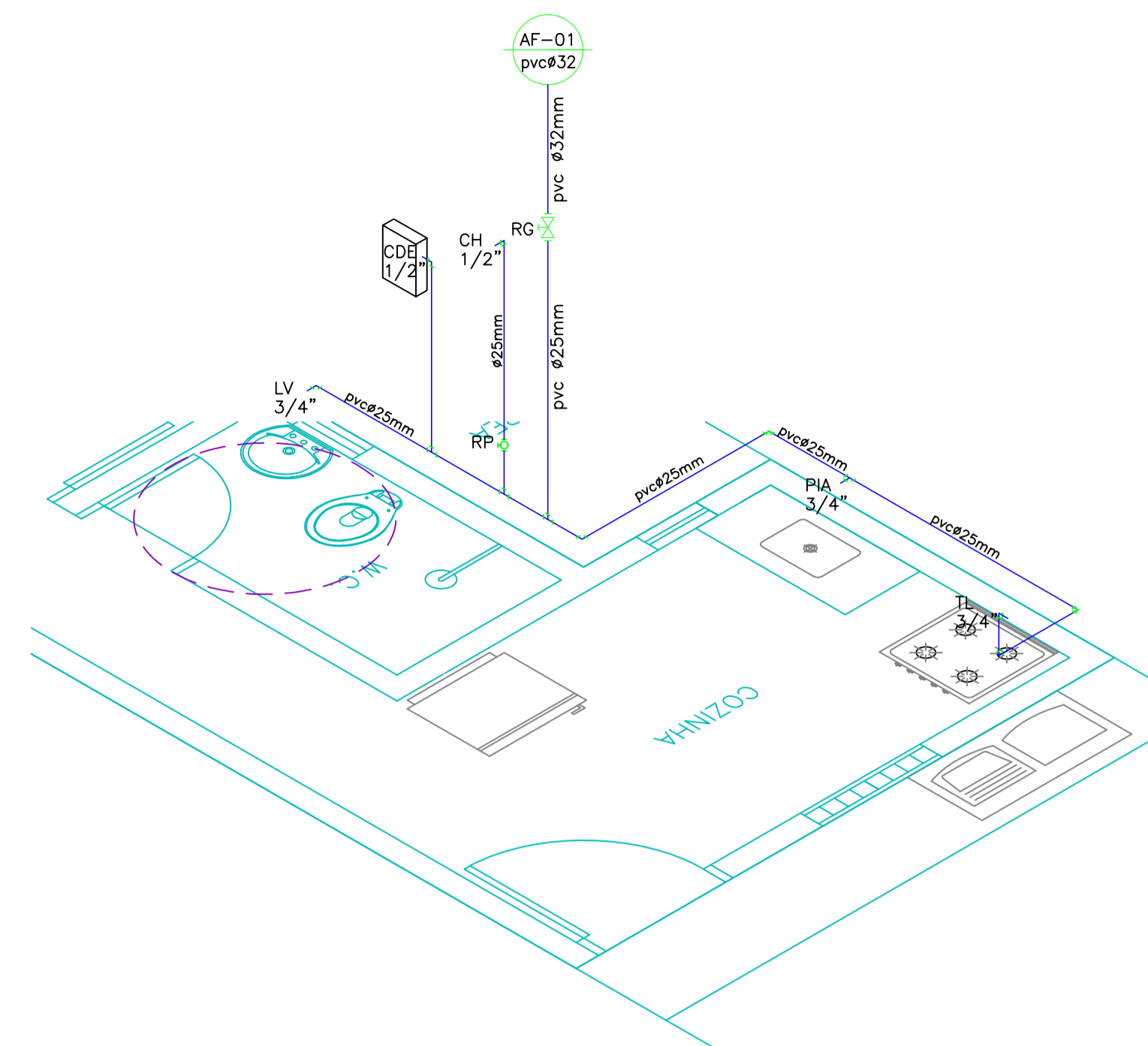
DETALHE ISOMÉTRICO ESC.: 1/25
