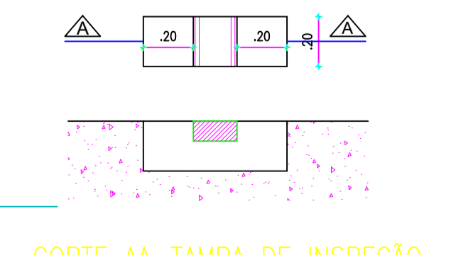
CORTE AA-TAMPA DE INSPEÇÃO ESCALA - 1:20
