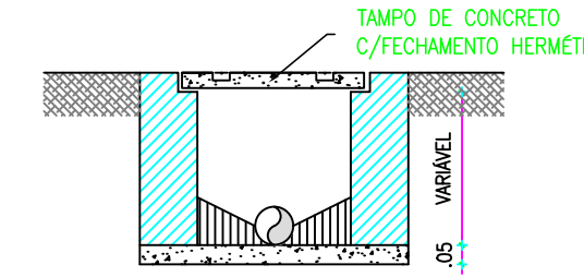
CORTE BB-TAMPA DE INSPEÇÃO ESCALA - 1:20
