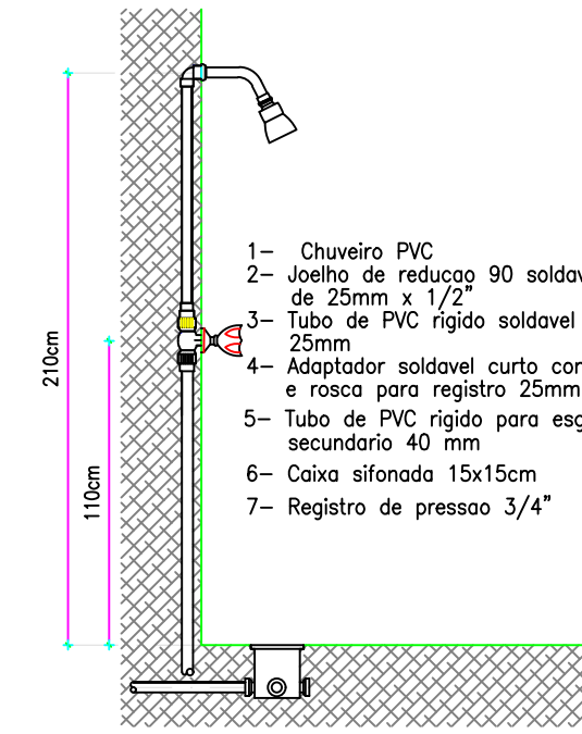
LIGAÇÃO CHUVEIRO
