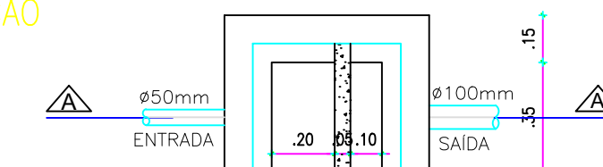
PLANTA BAIXA-CAIXA DE SABÃO ESCALA - 1:20
