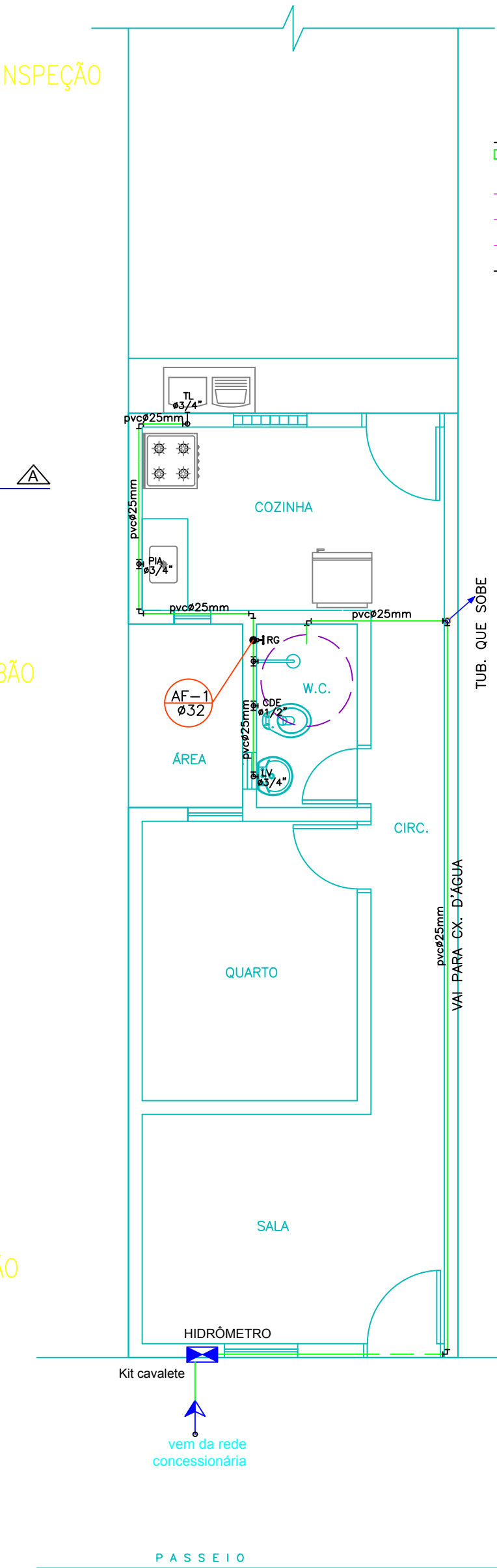
PLANTA BAIXA ESC.: 1/50
