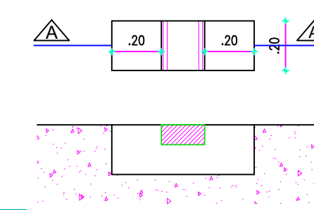
CORTE AA-TAMPA DE INSPEÇÃO ESCALA - 1:20
