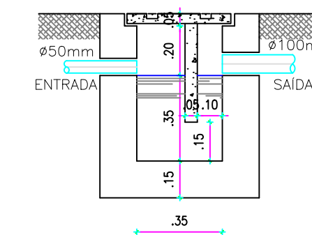
CORTE AA-CAIXA DE SABÃO ESCALA - 1:20
