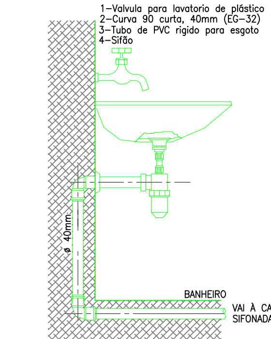
LIGAÇÃO LAVATÓRIO
