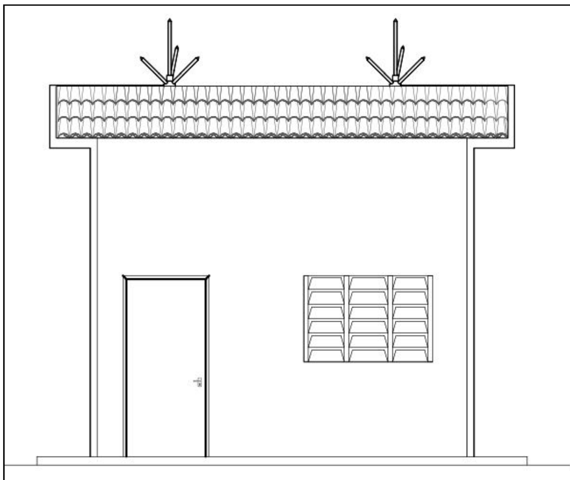
Fig. 1 - Detalhe dos captores
