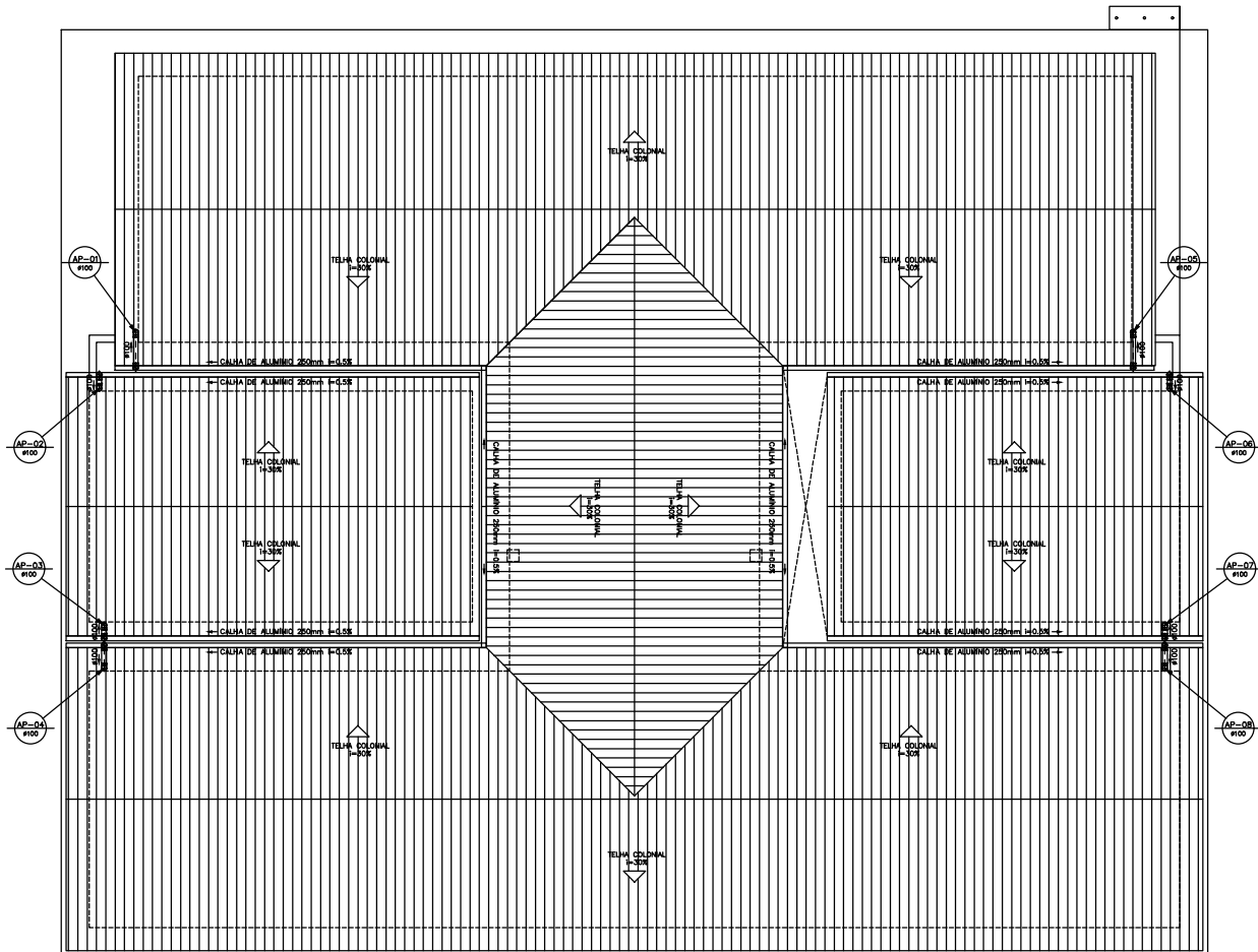
PLANTA COBERTA ESCALA _____ 1/50
