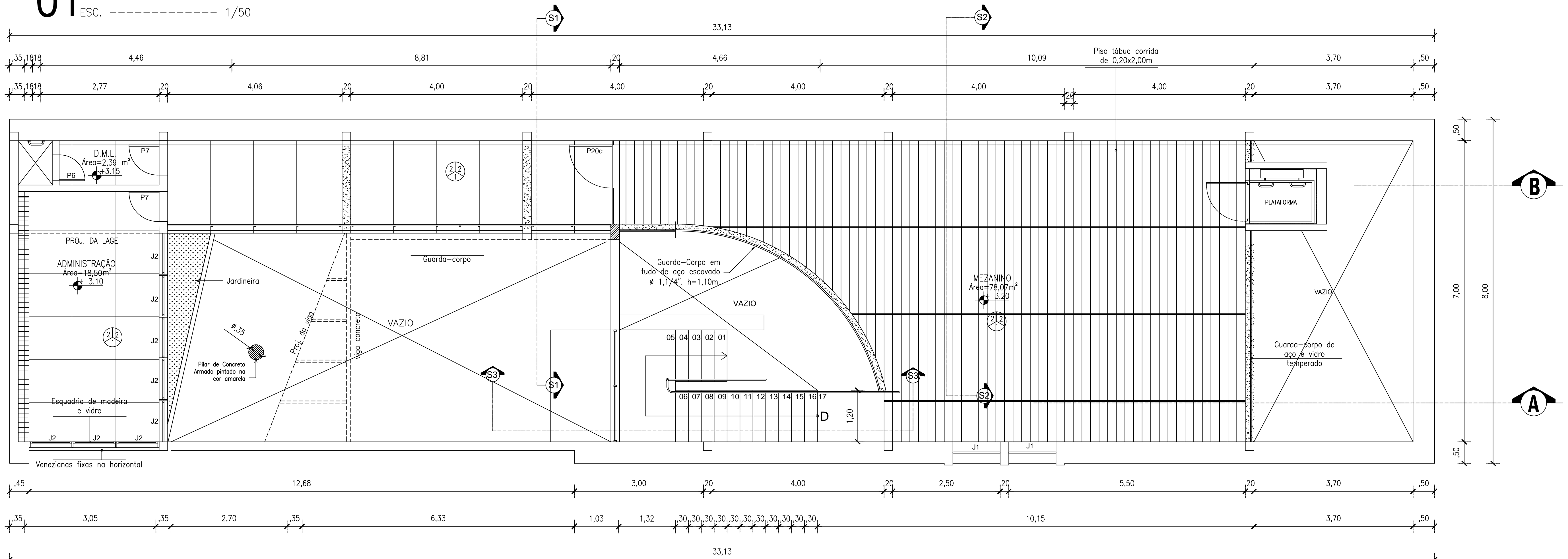
02 PLANTA BAIXA PAV.SUPERIOR ESC. ----- 1/50
