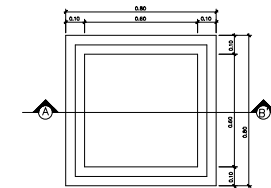
PLANTA BAIXA
