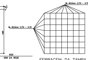
FERRAGEM DA TAMPA
