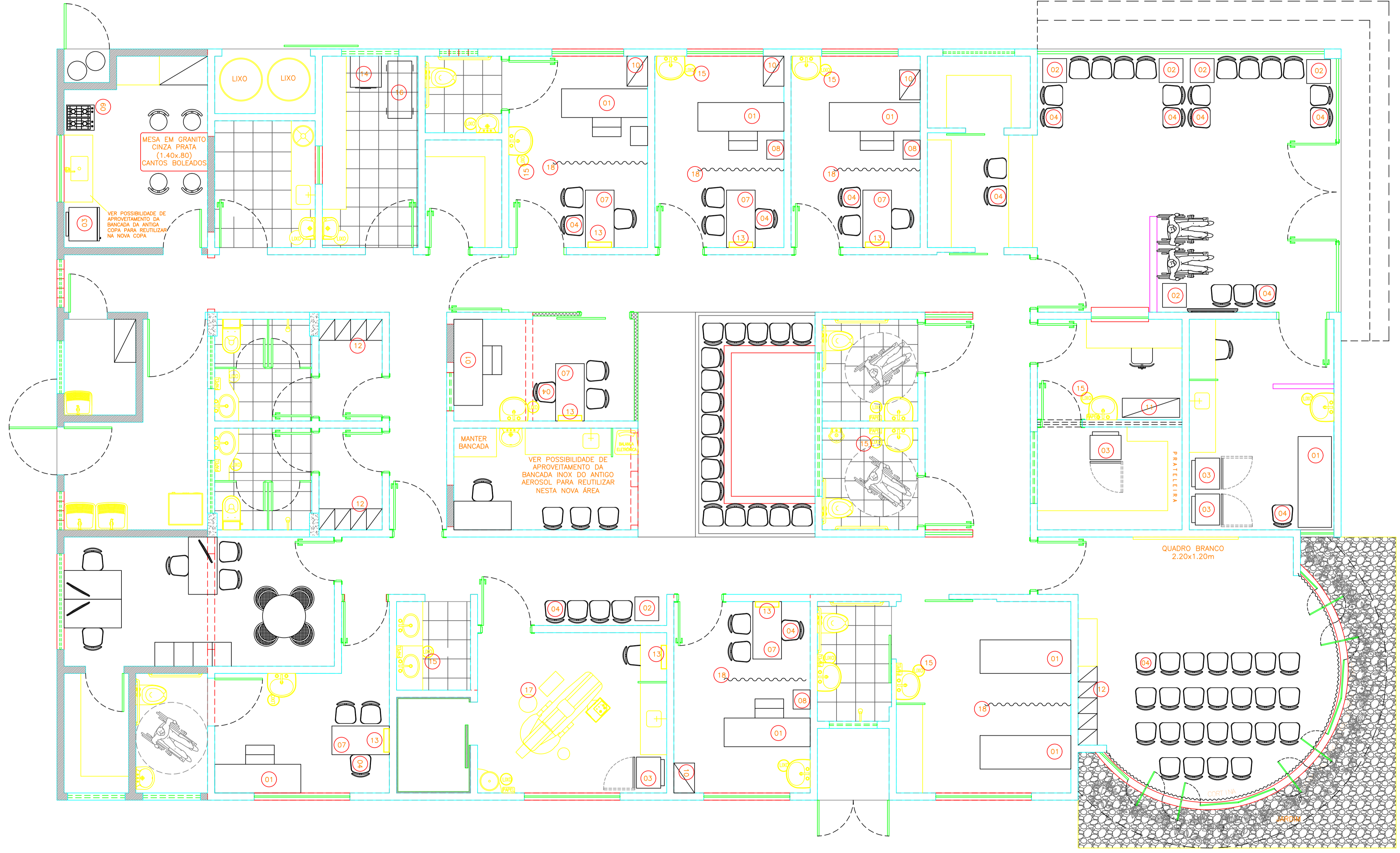
01 PLANTA BAIXA- LAYOUT esc: 1/50
