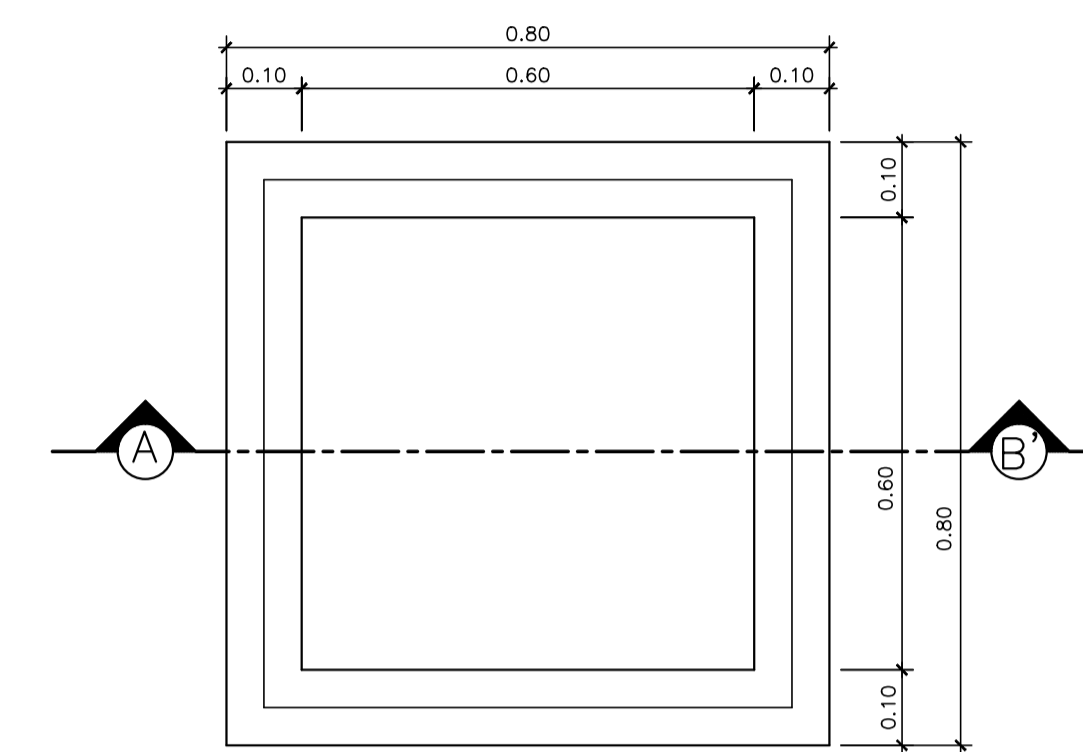
PLANTA BAIXA
