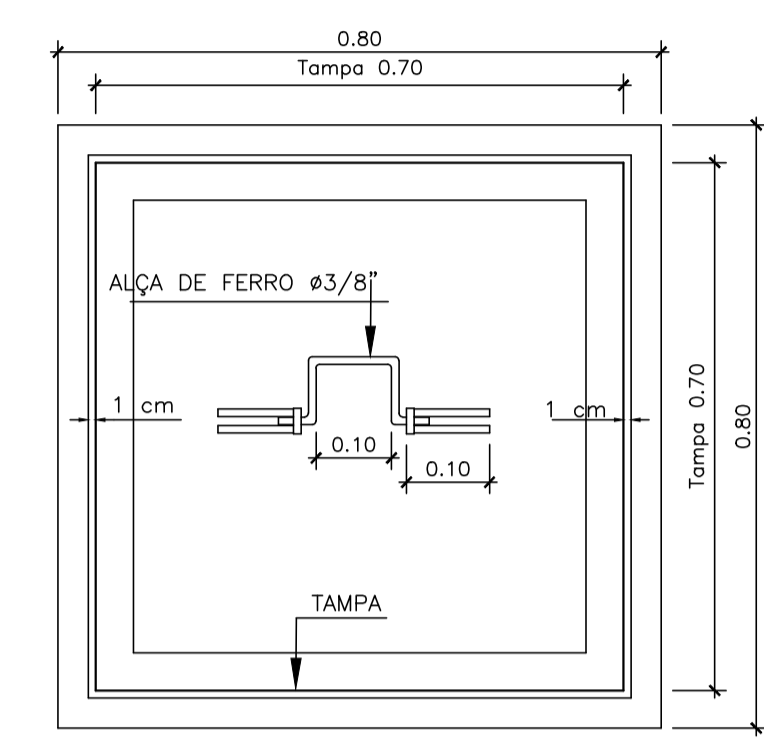
VISTA SUPERIOR.
