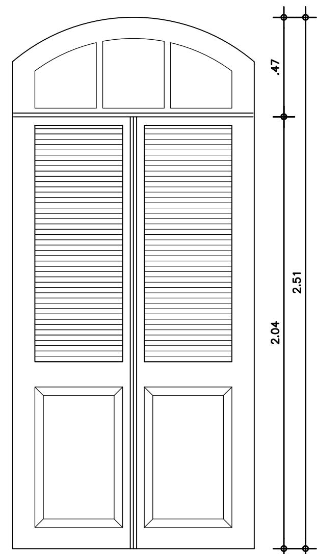
03 ELEVAÇÃO PORTA P14
