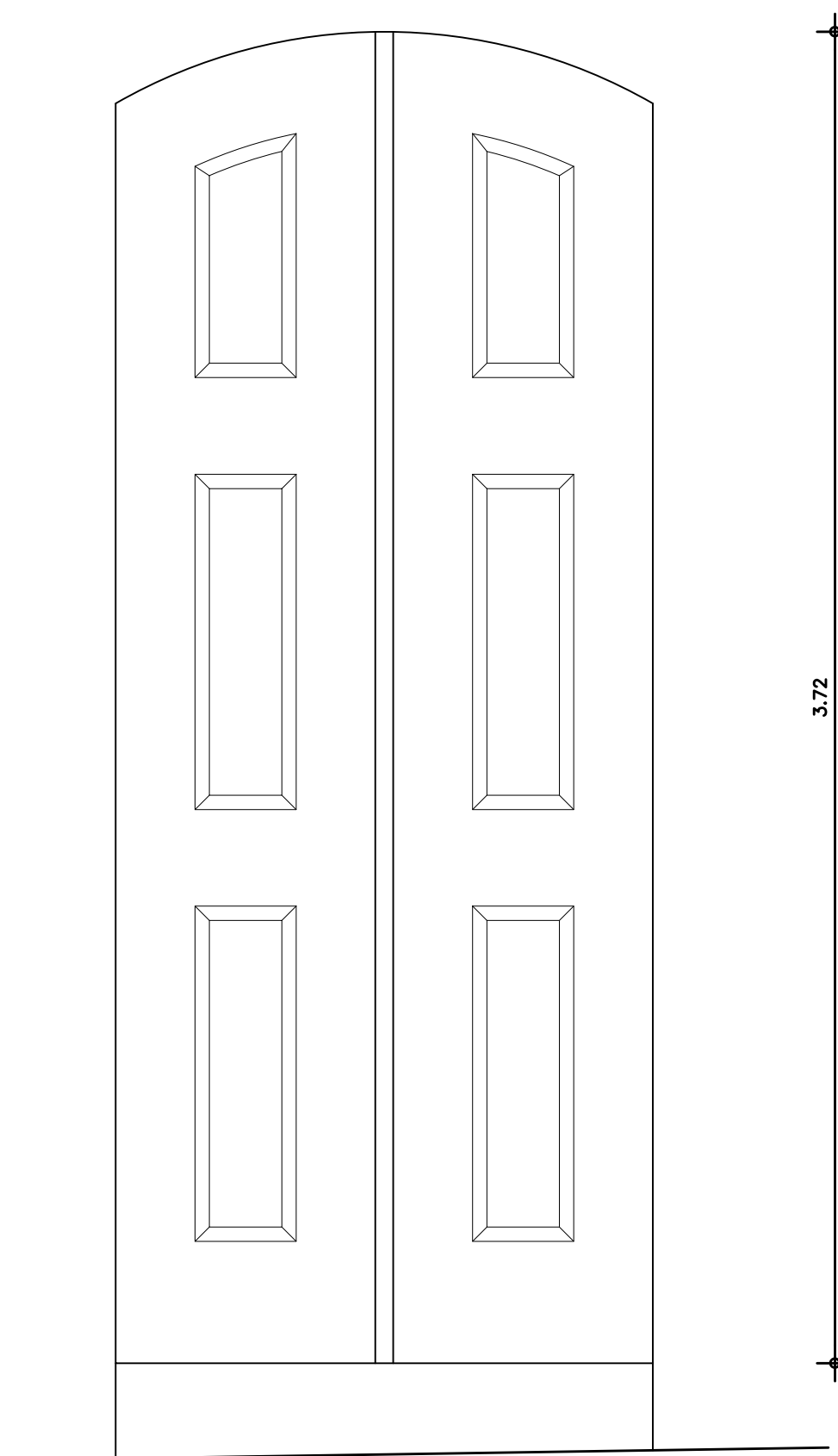
02 ELEVAÇÃO PORTA P1
