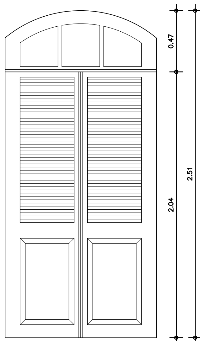
05 ELEVAÇÃO PORTA P16
