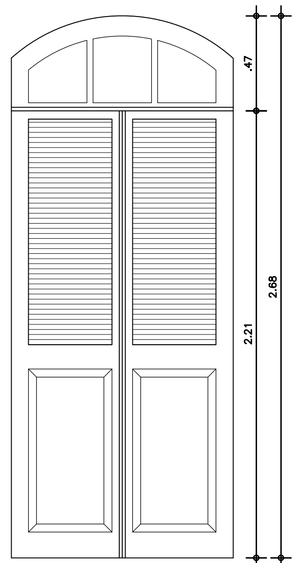
04 ELEVAÇÃO PORTA P15
