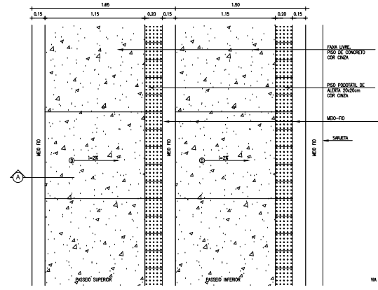
04 PLANTA BAIXA - CALÇADA DUPLA ESCALA — 1 : 20
