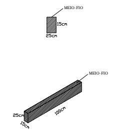
06 DET. MEIO-FIO ESCALA — 1 : 20
