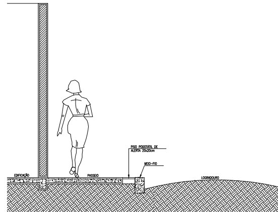
02 CORTE AA - CALÇADA SIMPLES ESCALA — 1 : 20
