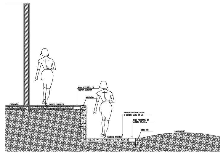
03 CORTE AA - CALÇADA SIMPLES ESCALA — 1 : 20
