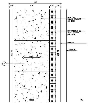
01 PLANTA BAIXA - CALÇADA SIMPLES ESCALA — 1 : 20
