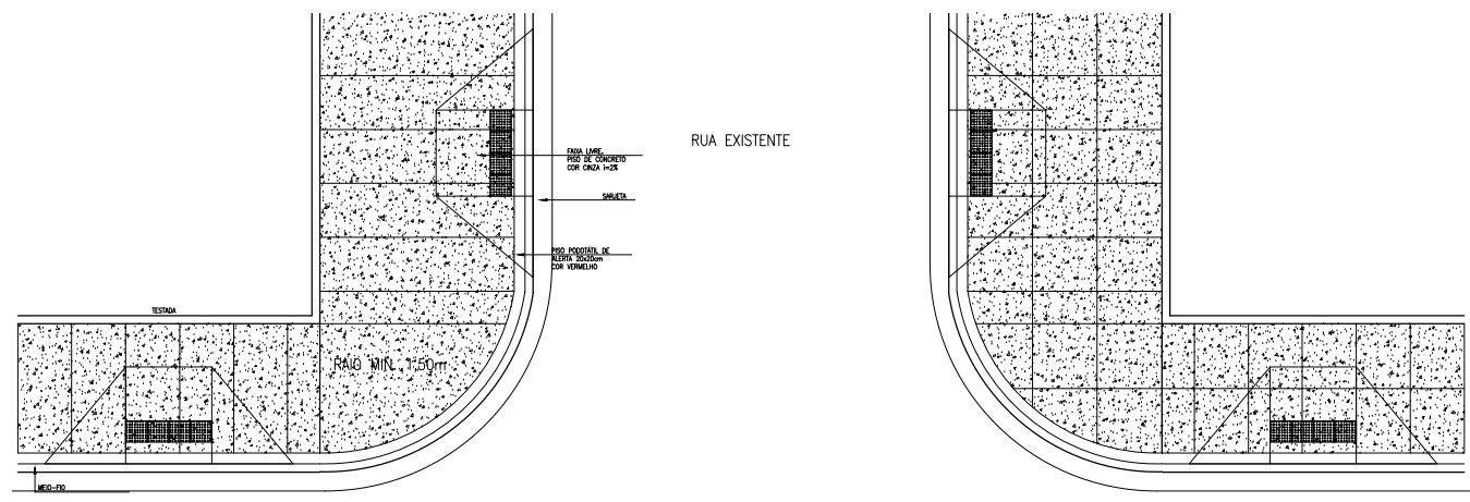
04 PLANTA BAIXA - CALÇADA DUPLA ESCALA — 1 : 20
