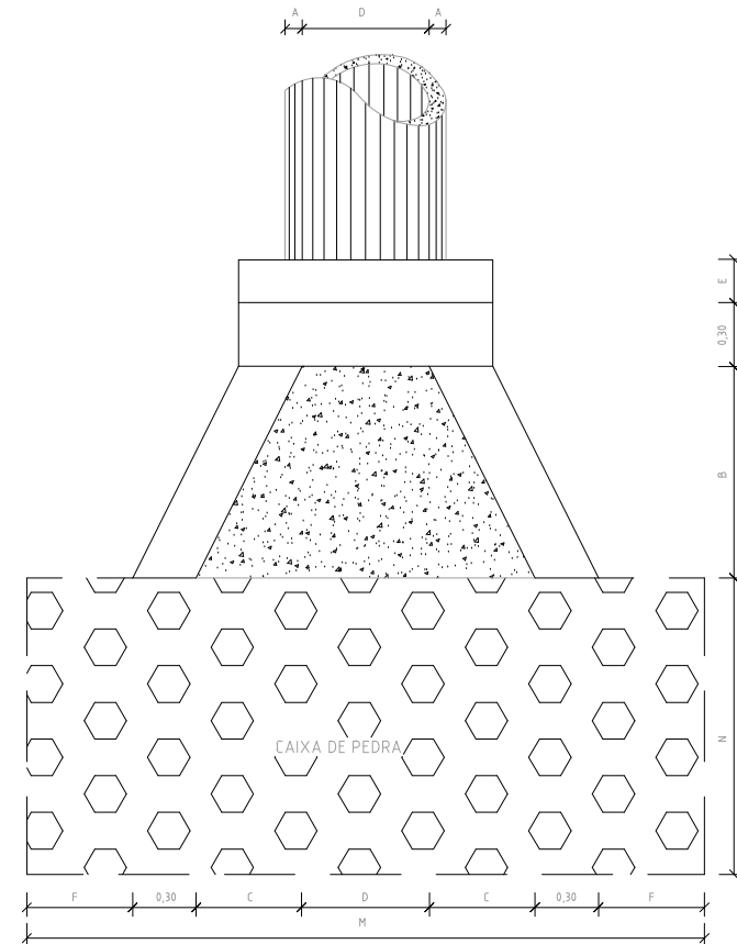
PROJEÇÃO HORIZONTAL
