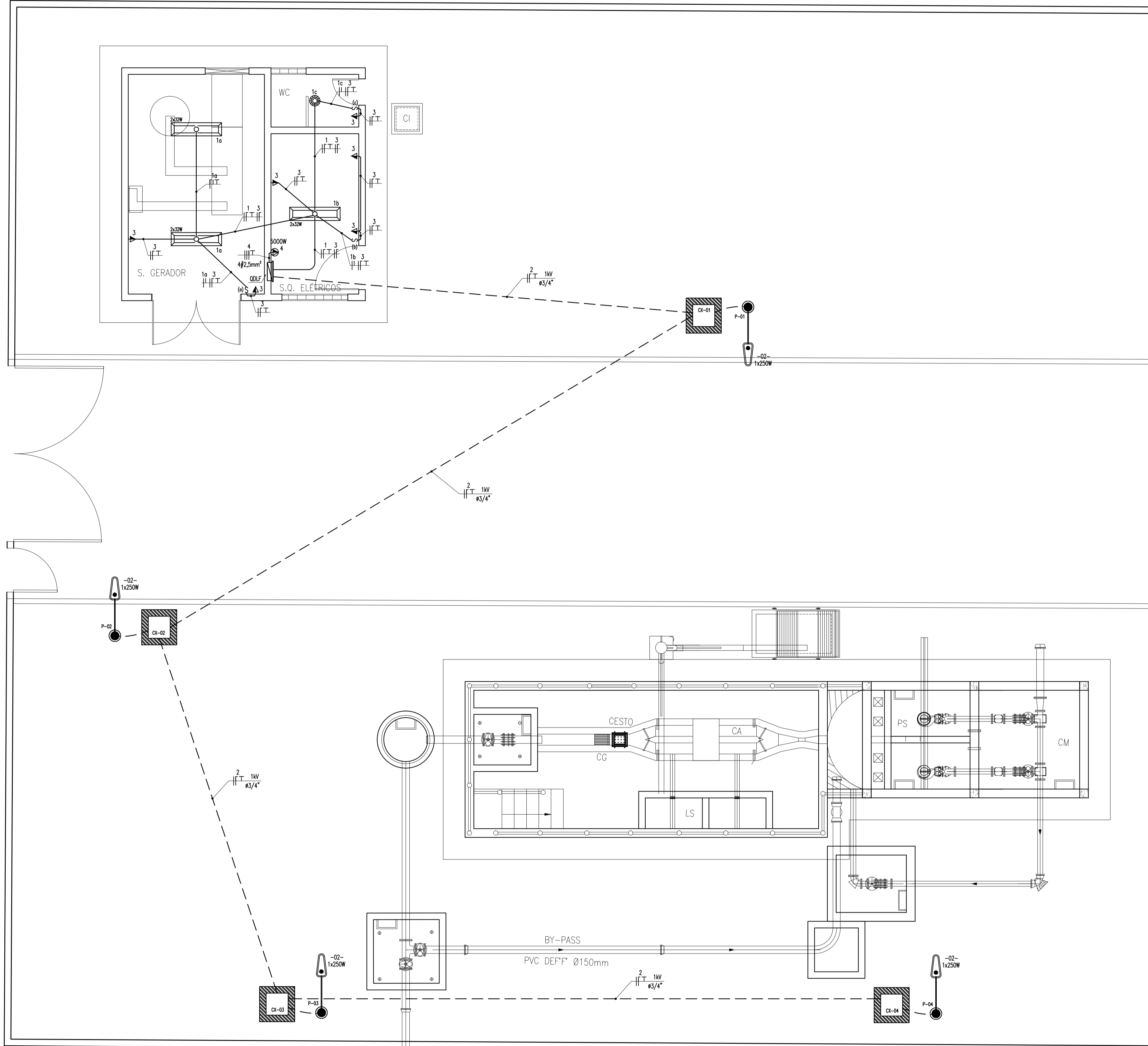
PLANTA BAIXA-ILUM INT E EXT Escala 1/50
