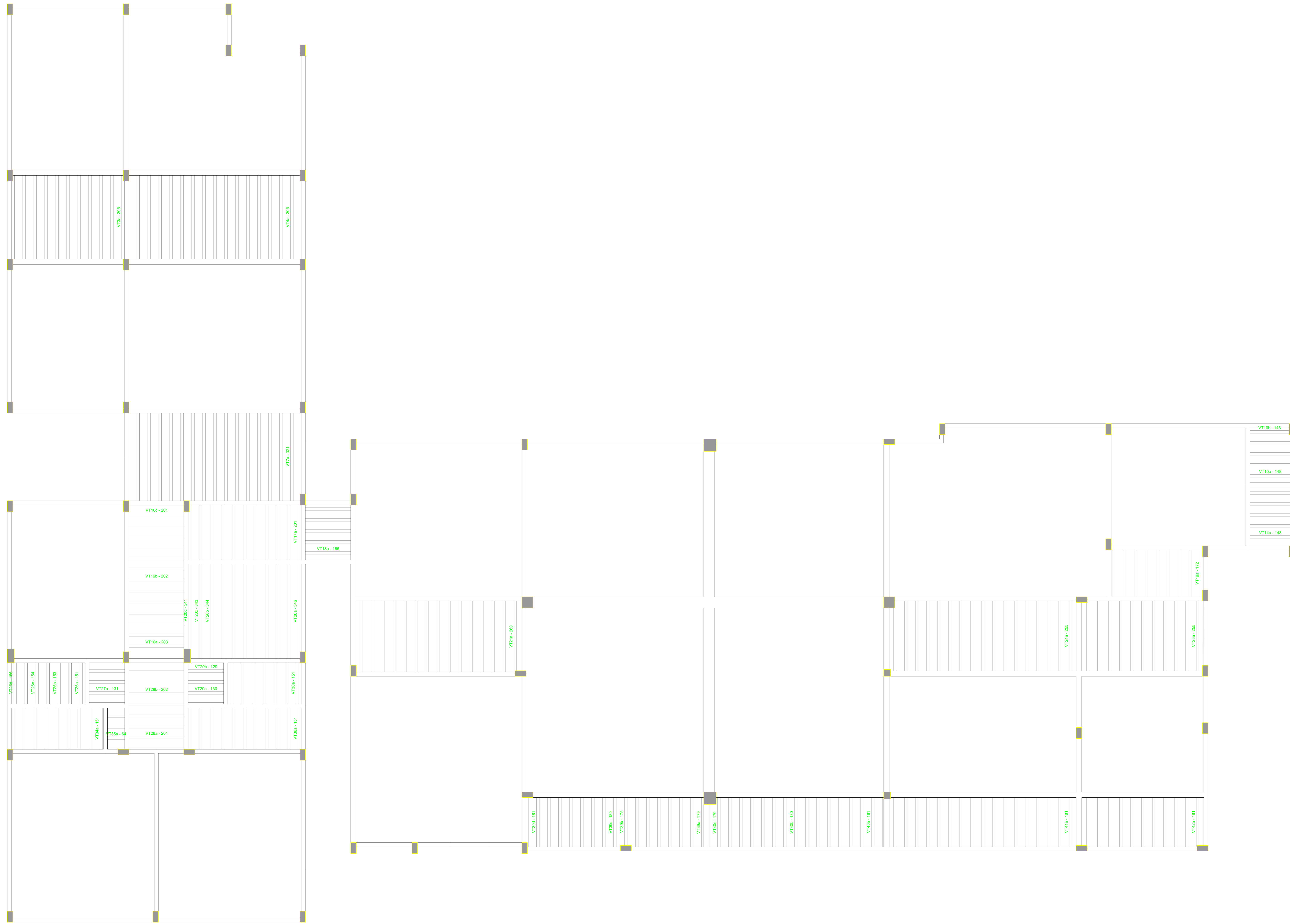
Planta de vigotas pré-moldadas escala 1:50
