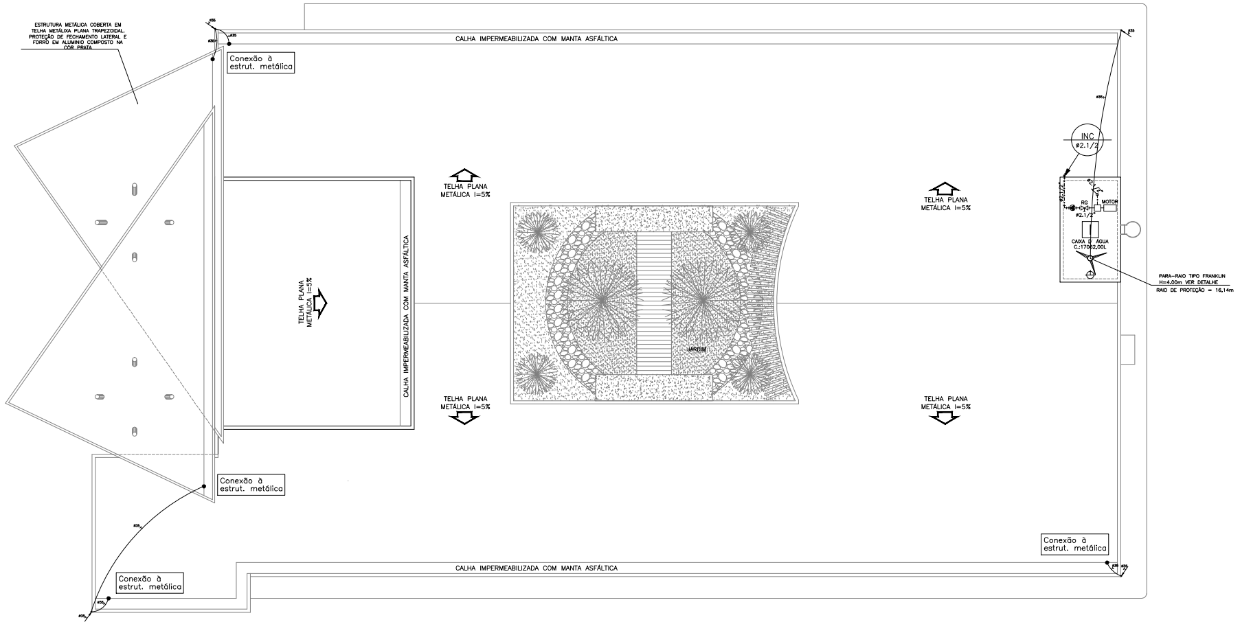
PLANTA DE COBERTA ESCALA 1/75
