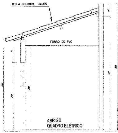
2 CORTE AA ESCALA: 1/25
