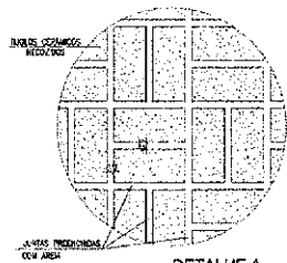
4 DETALHE A ESCALA: 50x
