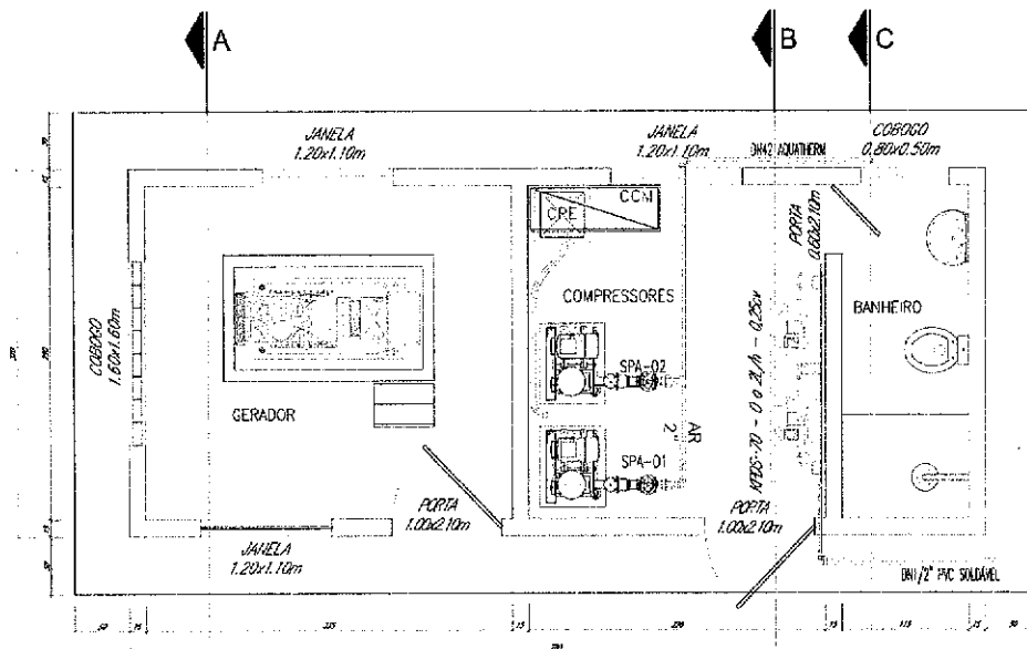
1 PLANTA BAIXA ESCALA: 1/25
