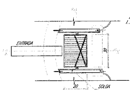
GRADE TIPO CESTO - PLANTA SEM ESCALA
