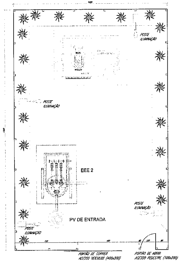
1 PLANTA URBANIZAÇÃO ESCALA: 1:50
