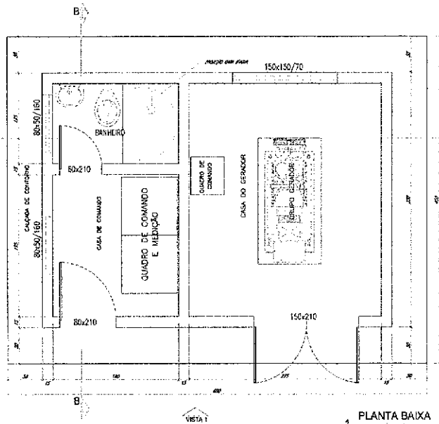
1 PLANTA BAIXA ESCALA: 1/25
