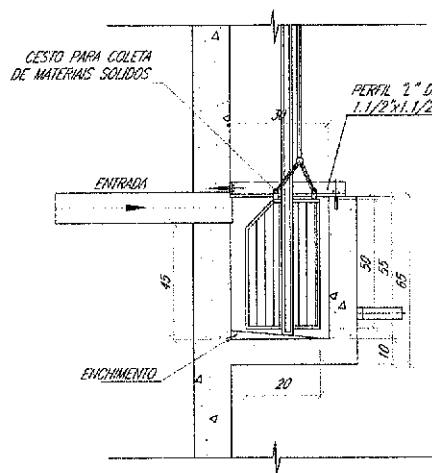
CORTE A-A SEM ESCALA
