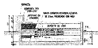
3 CORTE BB ESCALA: 1/50
