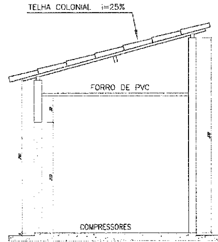
3 CORTE BB ESCALA: 1/25
