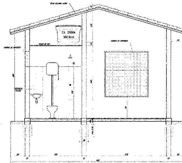
2 CORTE AA ESCALA: 1/25
