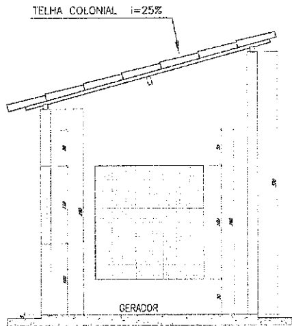
2 CORTE AA ESCALA: 1/25
