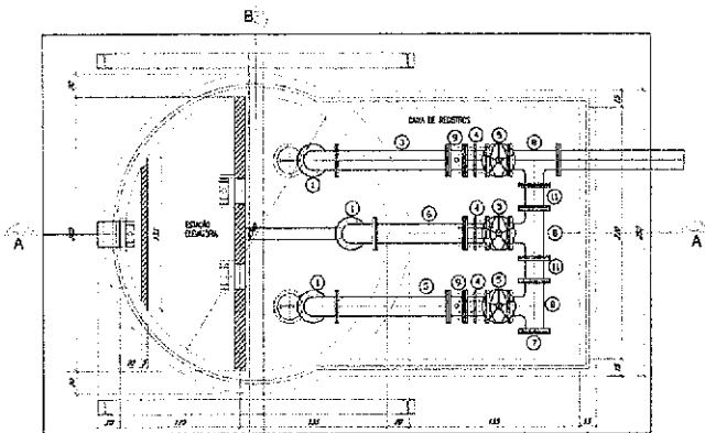
1 PLANTA BAIXA ESCALA: 1:25
