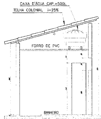
3 CORTE CC ESCALA: 1/25
