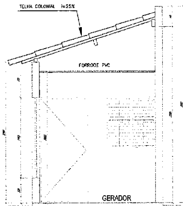
3 CORTE BB ESCALA: 1/25
