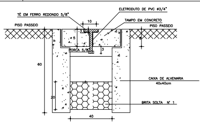
DETALHE CX. DE PASS. SEM ESCALA
