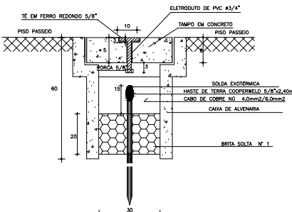
DETALHE ATERRAMENTO SEM ESCALA
