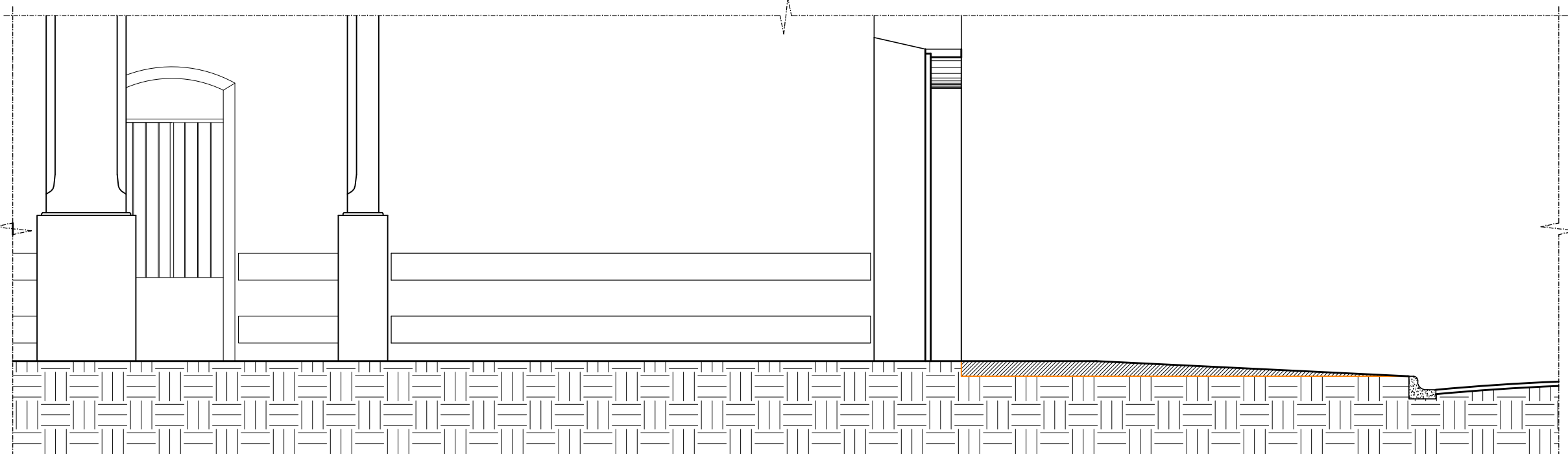
02 CORTE SETORIAL A' A' ESC. 1/75
