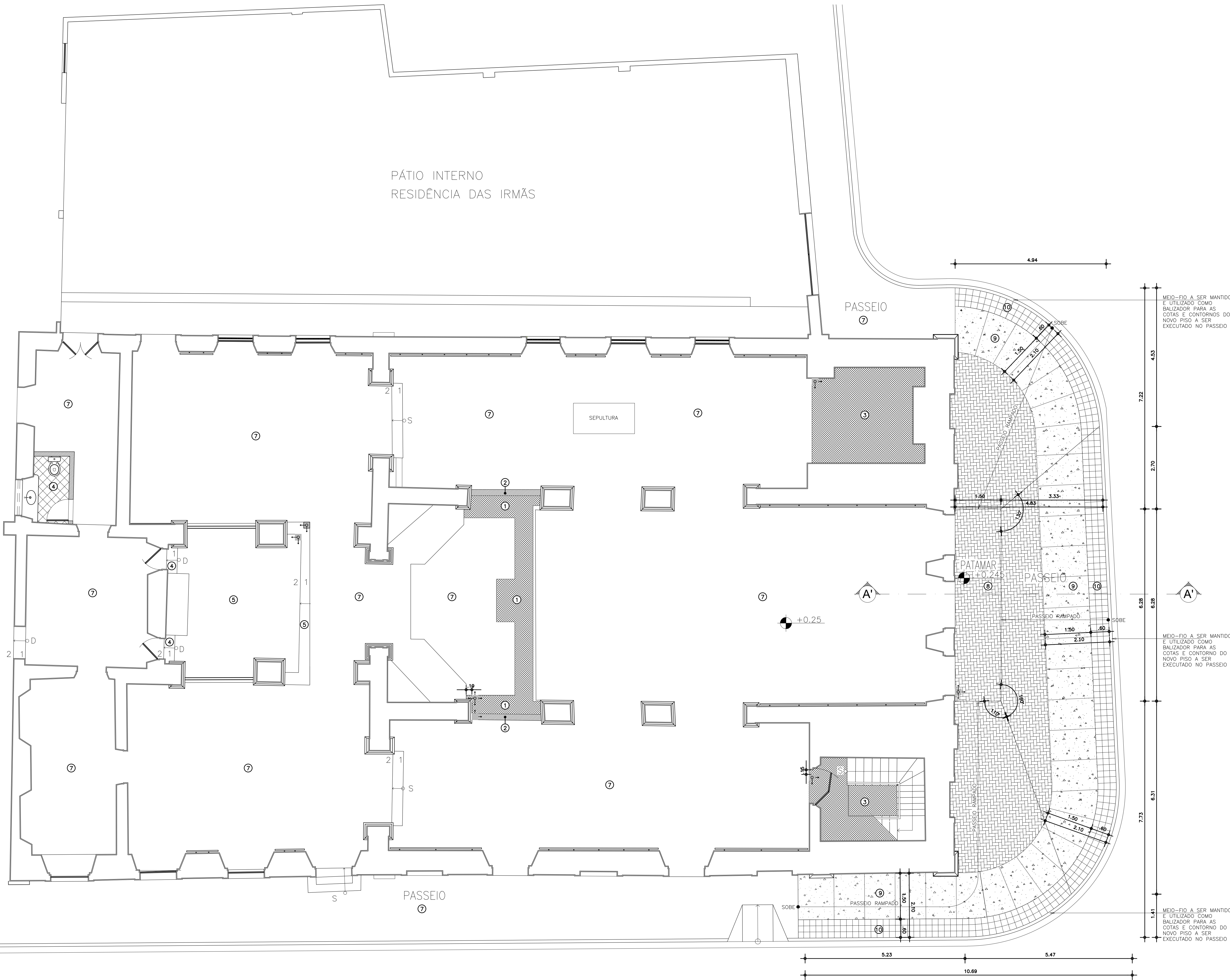
01 PLANTA PAGINAÇÃO DE PISO TÉRREO ESC. 1/75
