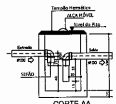
CORTE AA
