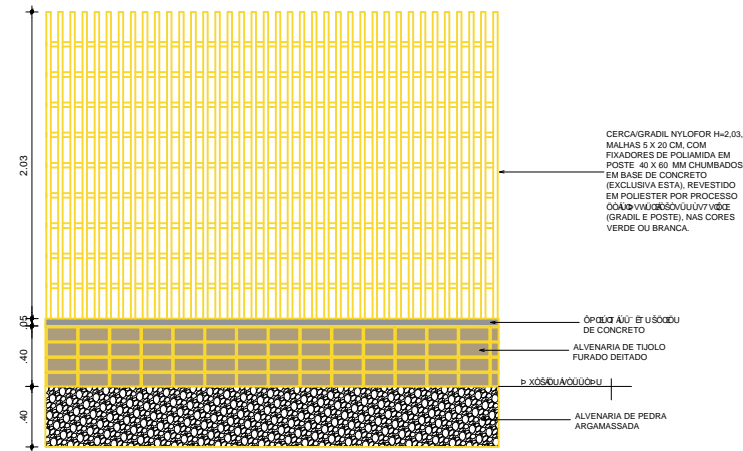
CORTE AA
