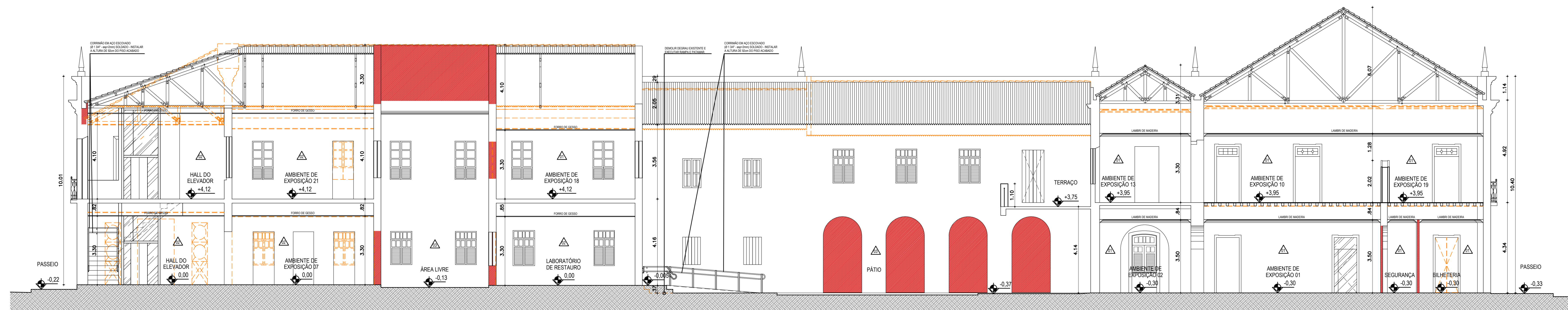
02 CORTE LONGITUDINAL AA PROJETO ARQUITETÔNICO ESCALA 1/75
