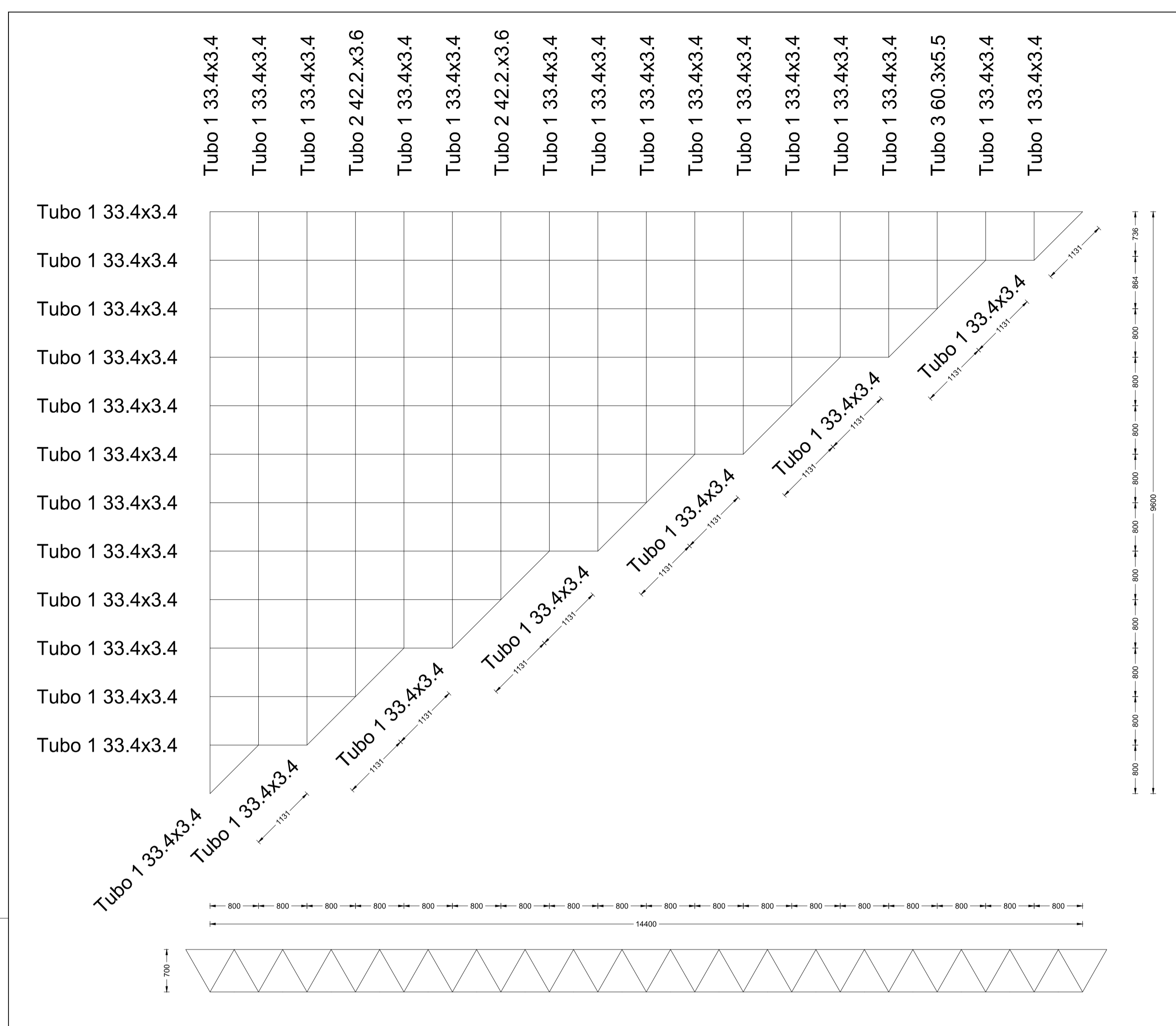
1 MALHA ESPACIAL 01 - INFERIOR ESCALA 1:50
