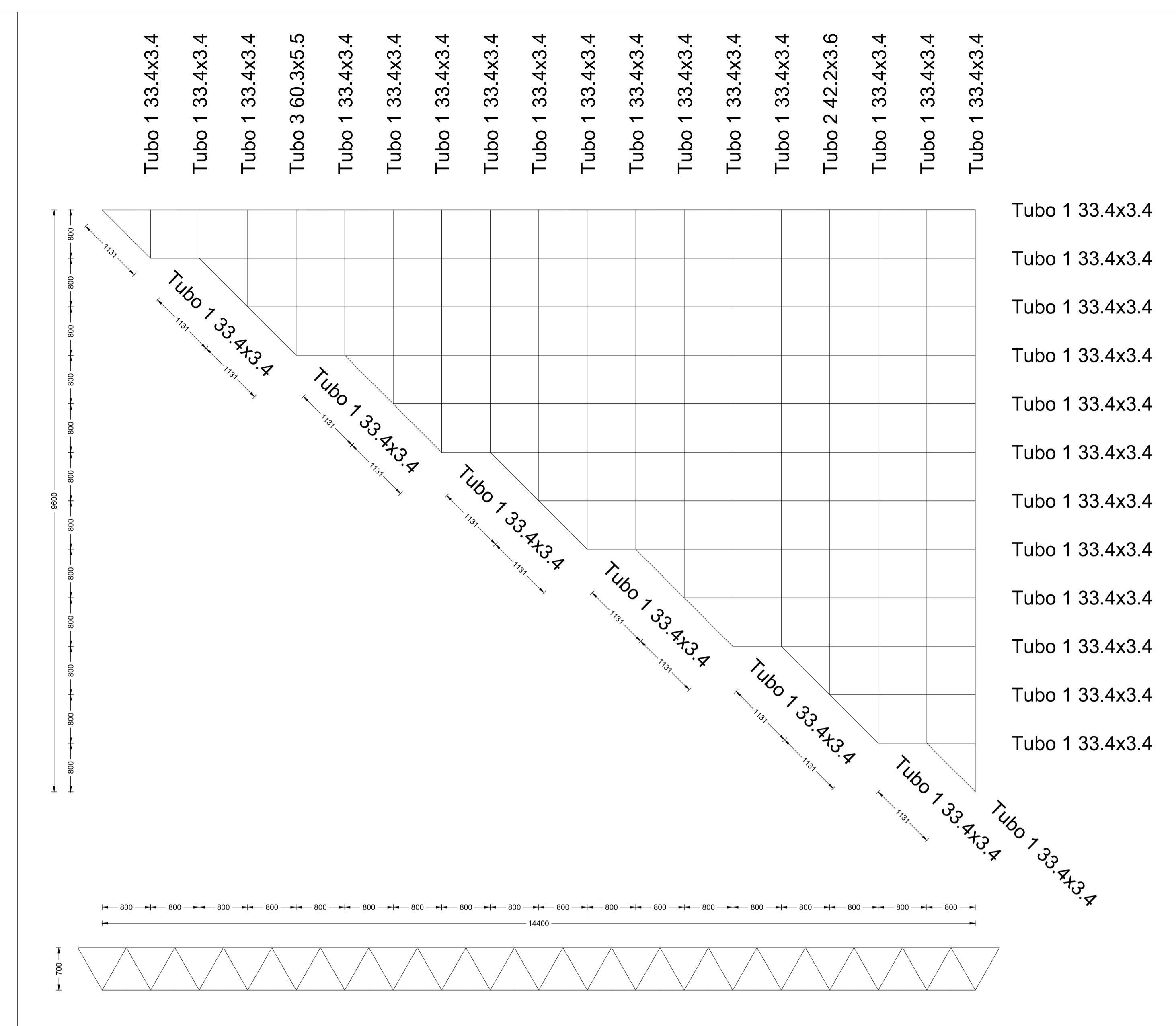
2 MALHA ESPACIAL 02 - INFERIOR ESCALA 1:50
