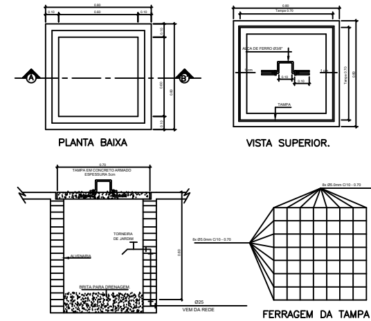
DETALHE EXECUTIVO DA CAIXA COM TORNEIRA DE JARDIM CAIXA DE PASSAGEM 60x60x60cm - TAMPA DE CONCRETO
