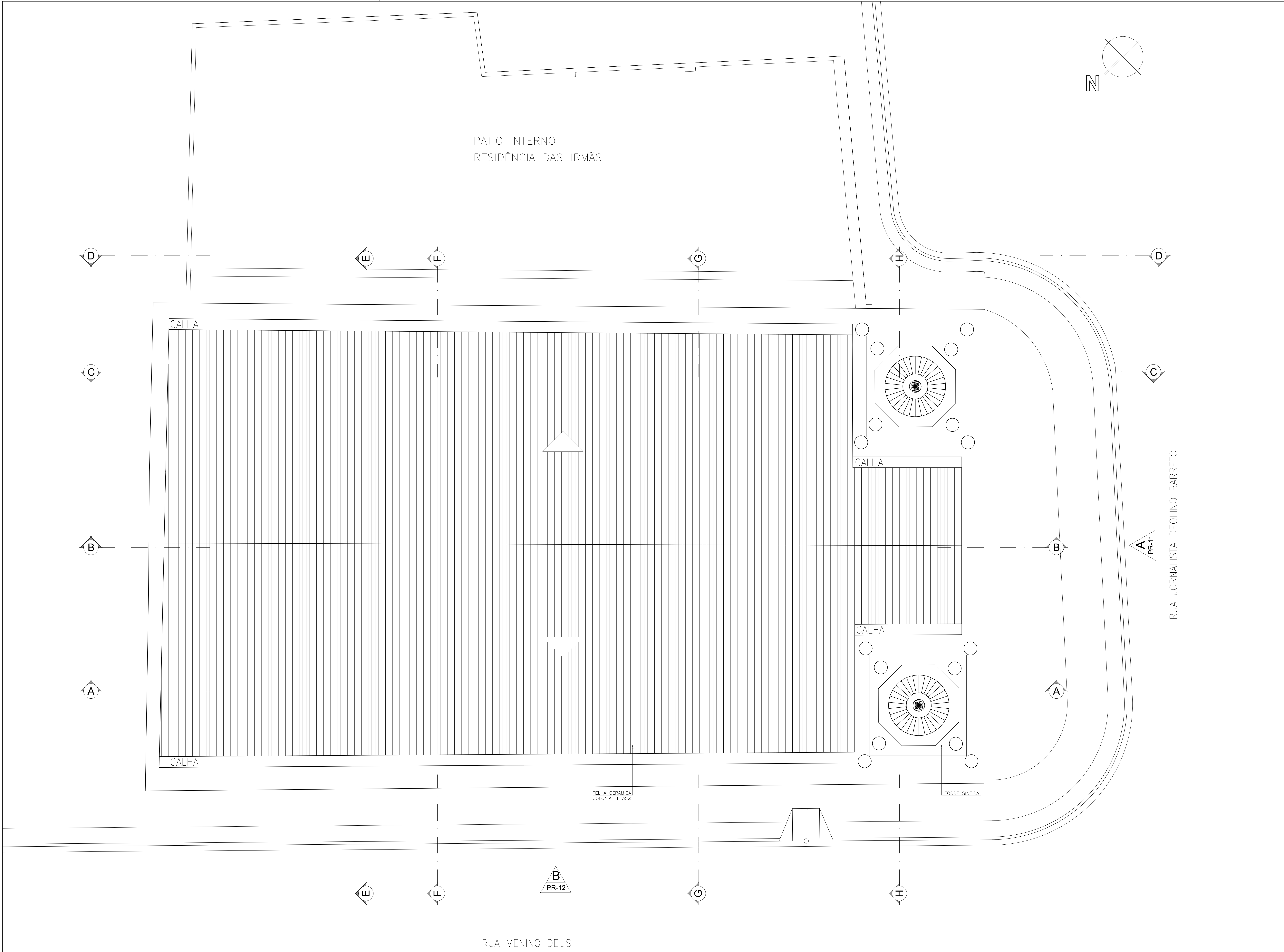
01 PLANTA DE COBERTA
