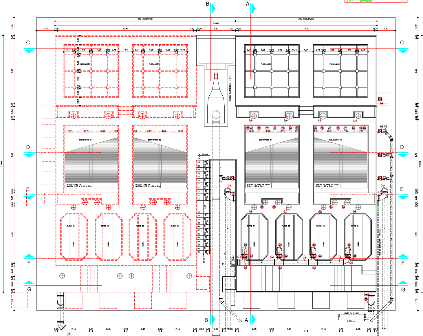
PLANTA BAIXA-NÍVEL 1 ESCALA = 1/50
