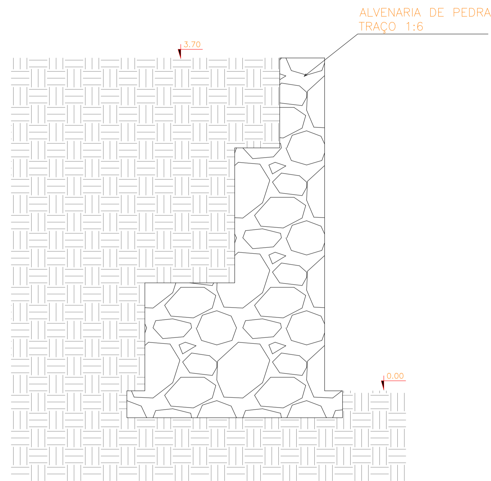
03 DETALHE - MURO 02 ESC.: 1/25
