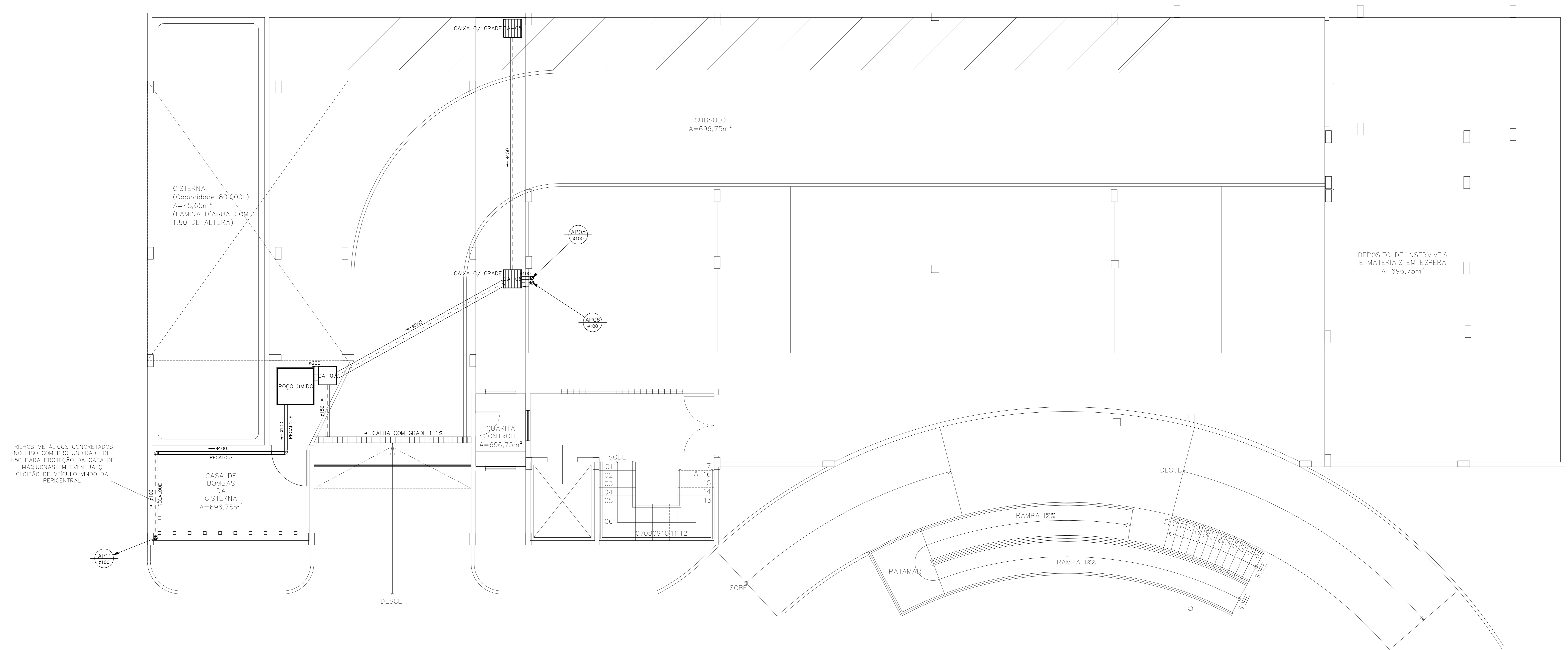
PLANTA BAIXA SUBSOLO ESCALA 1/50
