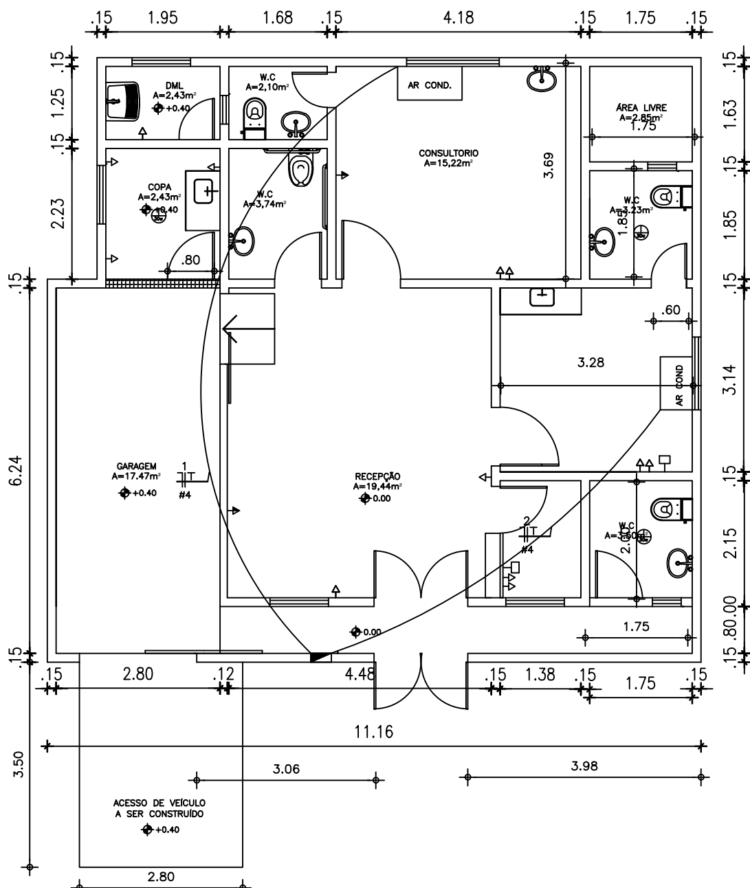
04 ELÉTRICO ESCALA - 1: 100
