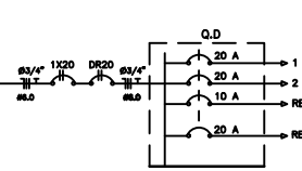
DIAGRAMA UNIFILAR ESCALA 1:100
