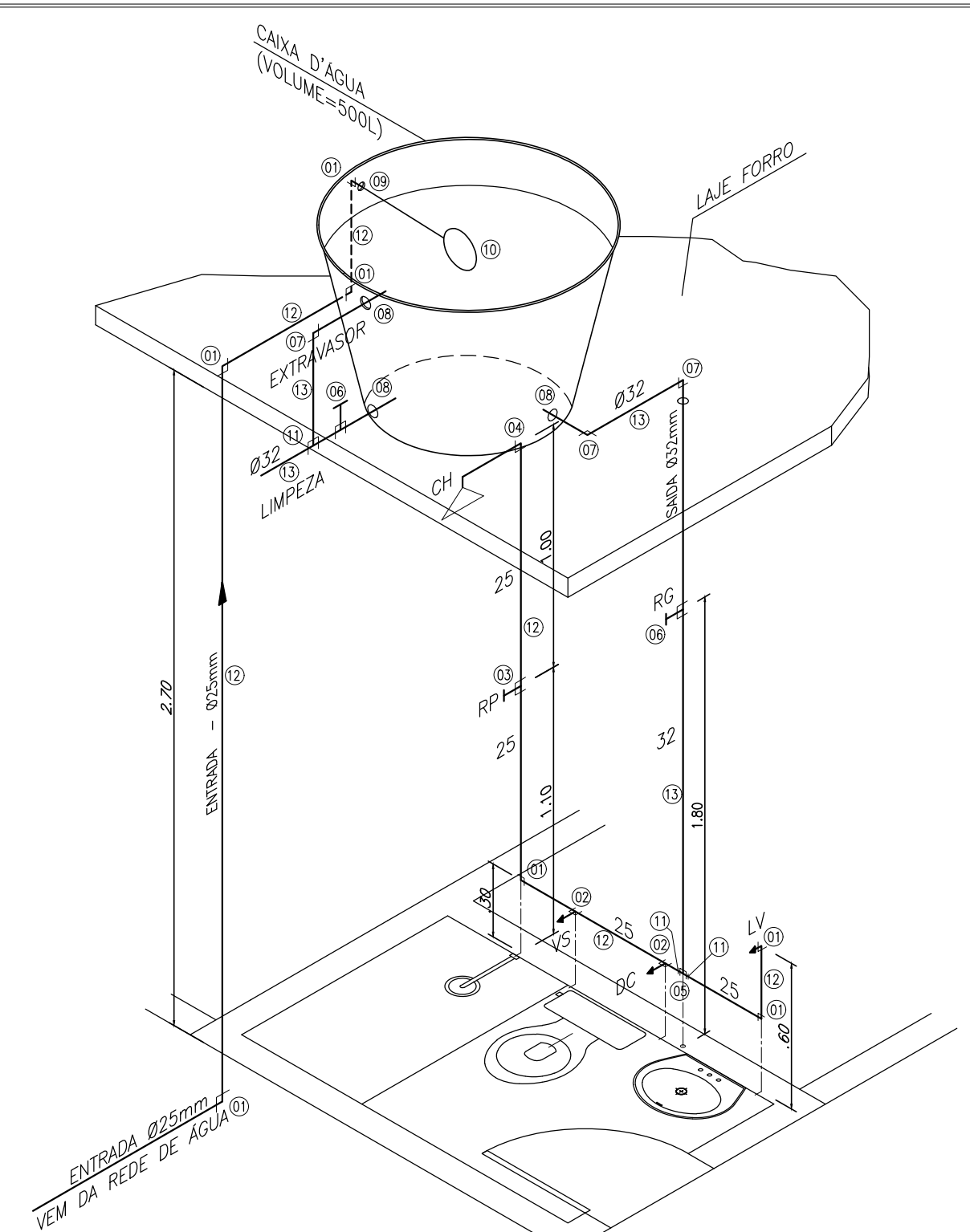
ISOMÉTRICO WC - INSTALAÇÃO HIDRÁULICA ESCALA 1:25
