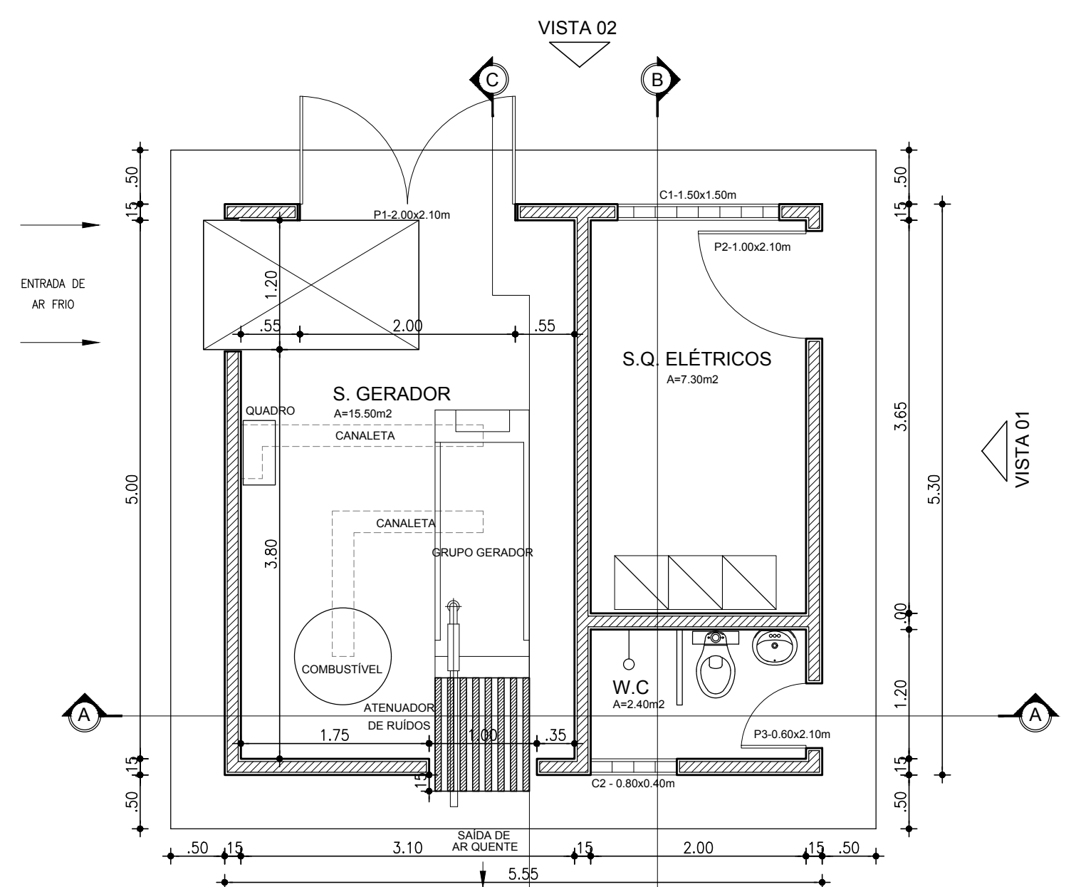
PLANTA BAIXA PLANO ESCALA 1:50
