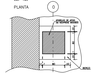
DETALHE - D1
