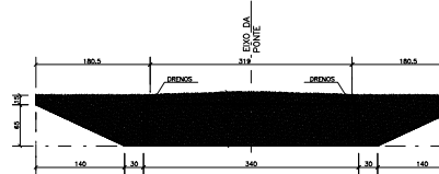
SEÇÃO TRANSVERSAL DO TABULEIRO (EIXO 0 a 1)
