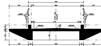
SEÇÃO TRANSVERSAL DO TABULEIRO (EIXO 1 ao 7)
