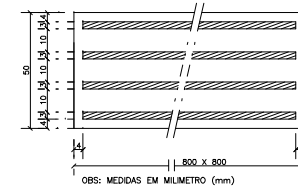
DETALHE APARELHO DE APOIO DE NEOPRENE
