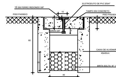
DETALHE CX. DE PASS. SEM ESCALA
