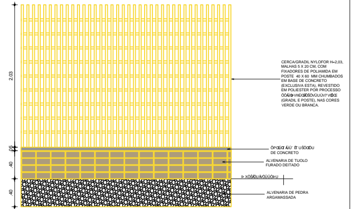
2 DETALHAMENTO DE GRADIL - CORTE LONGITUDINAL SEM ESCALA
