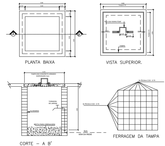
DETALHE EXECUTIVO DA CAIXA COM TORNEIRA DE JARDIM CAIXA DE PASSAGEM 60x60x60cm – TAMPA DE CONCRETO
