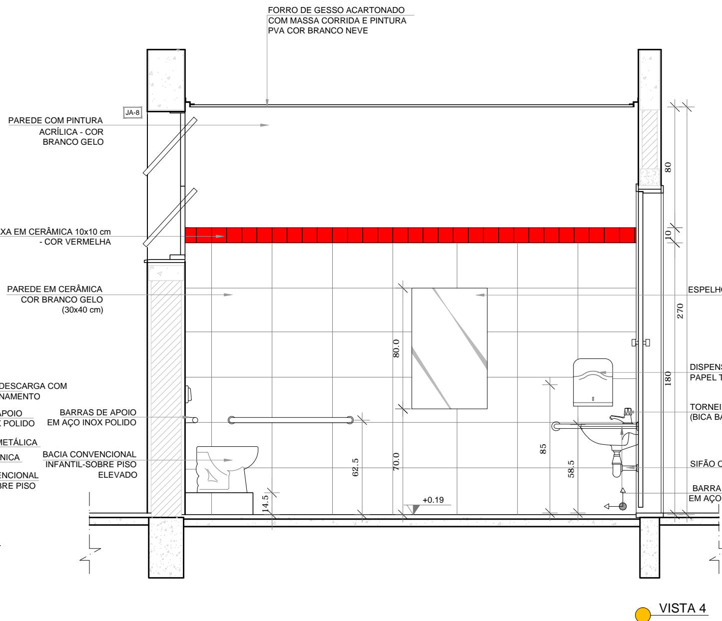
VISTA 4
