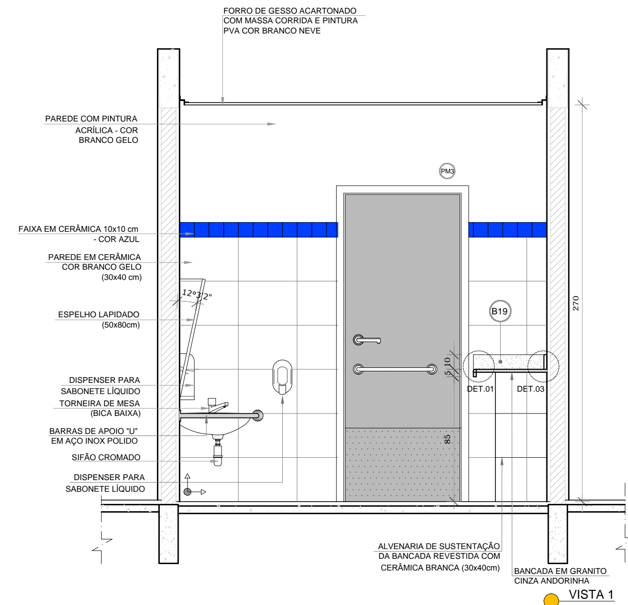
VISTA 1
