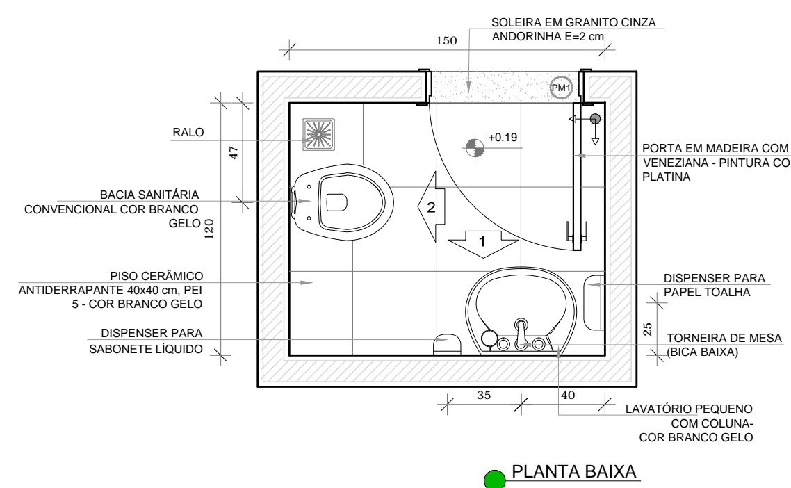
PLANTA BAIXA
