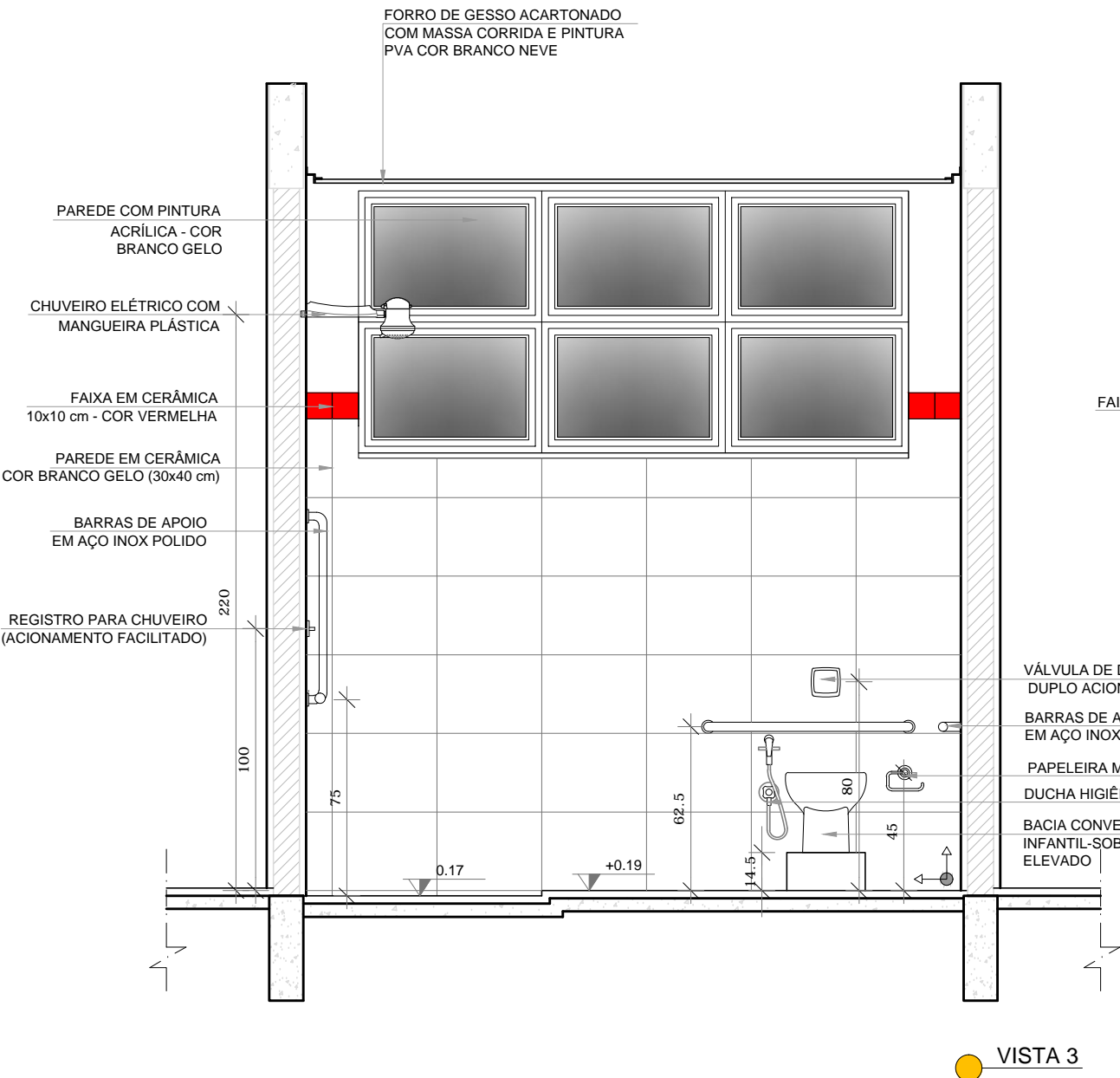
VISTA 3
