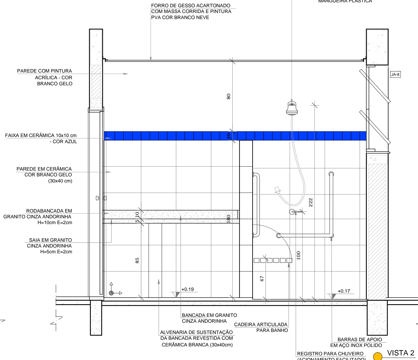
VISTA 2
