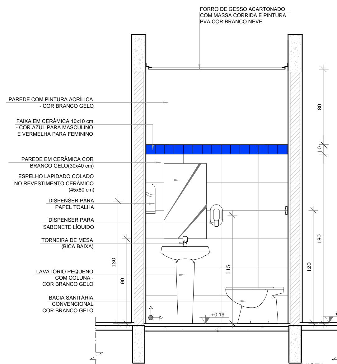
VISTA 1
