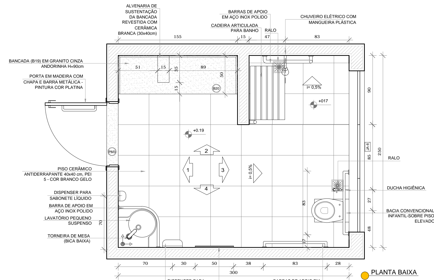
PLANTA BAIXA
