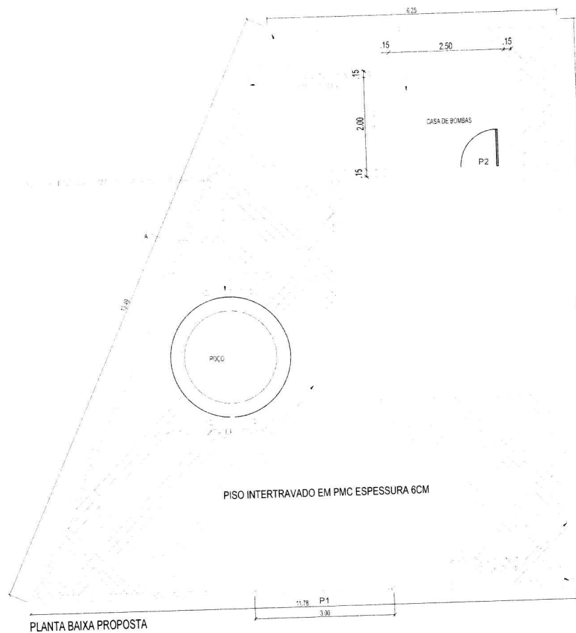
PLANTA BAIXA PROPOSTA
