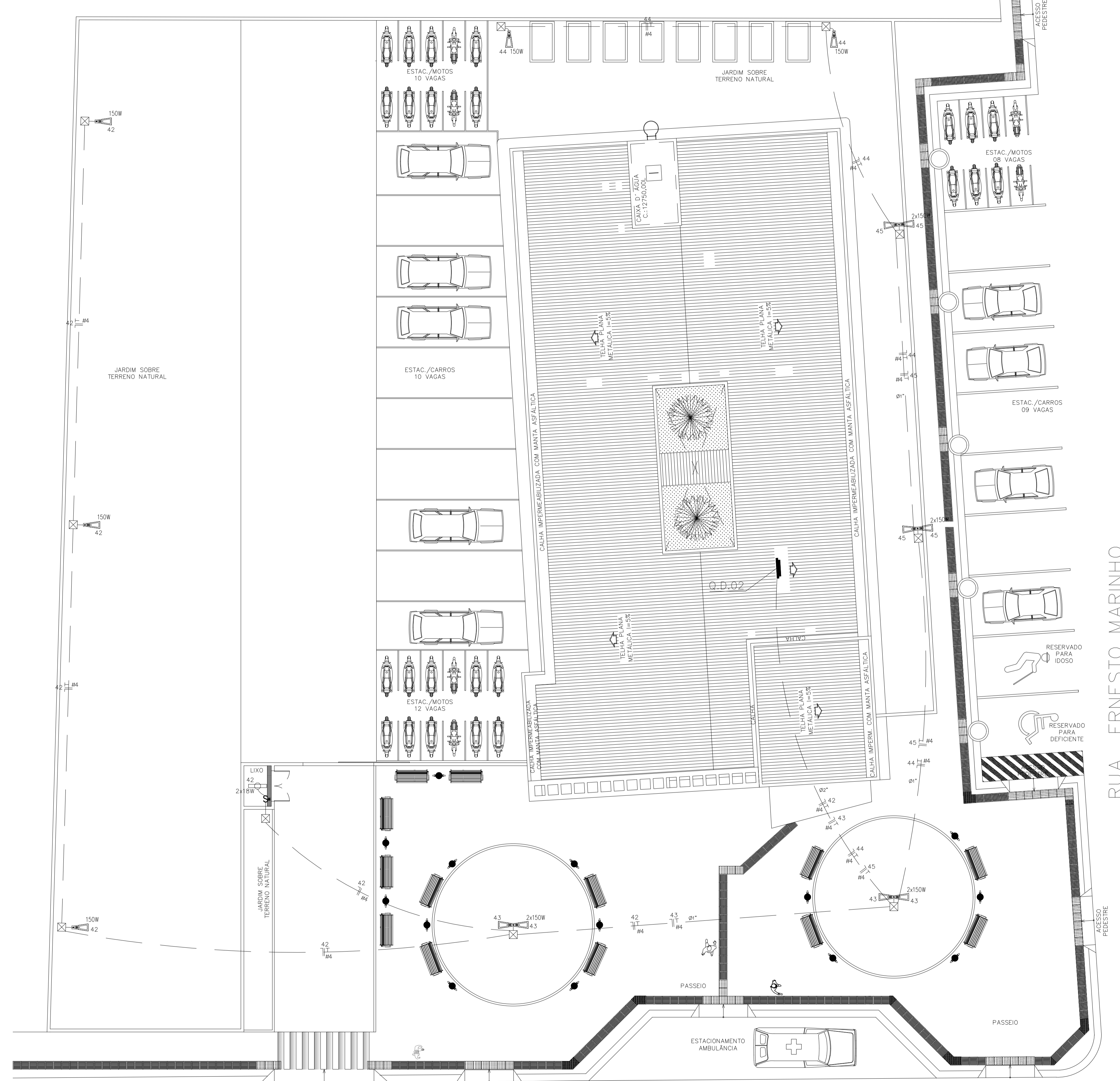
PLANTA BAIXA IMPLANTAÇÃO ESCALA 1/100
