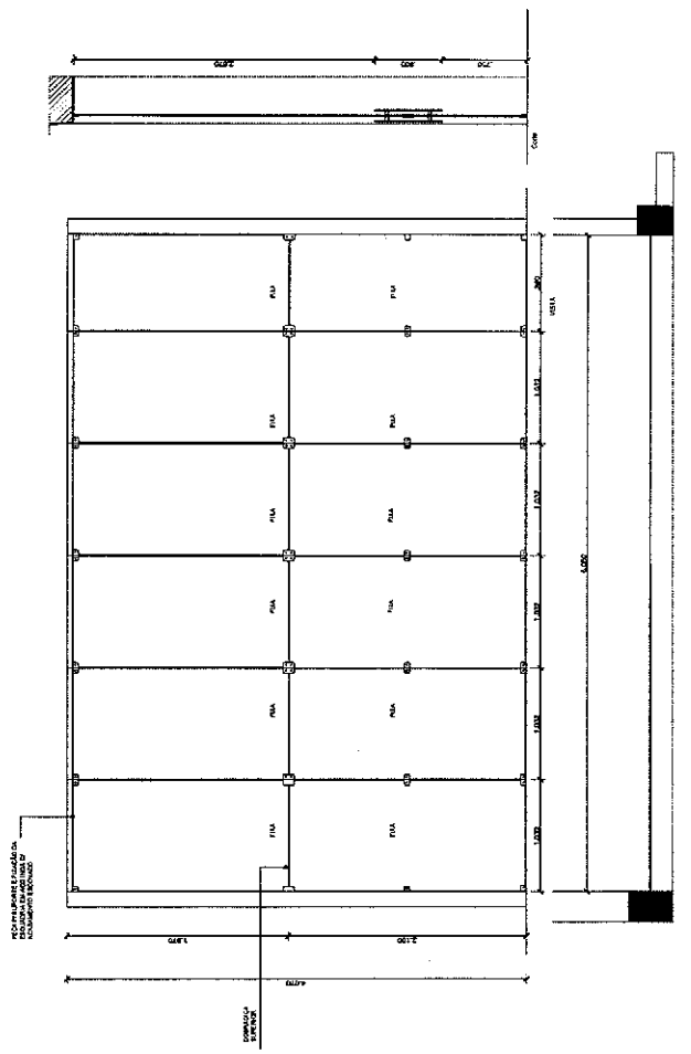
02 Esquadria P/07
