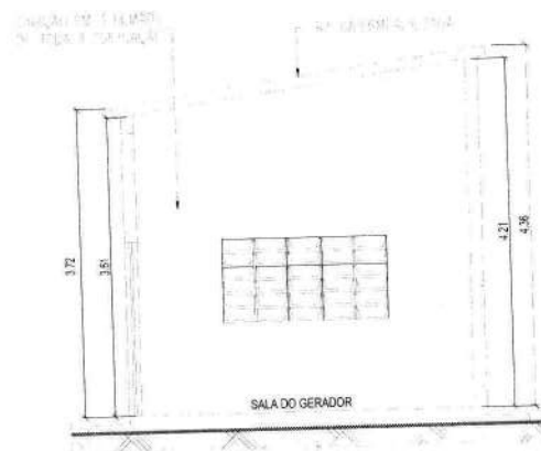
CORTE A-A
