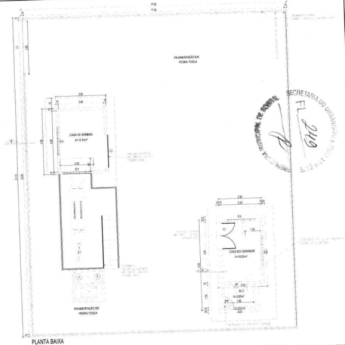
PLANTA BAIXA
