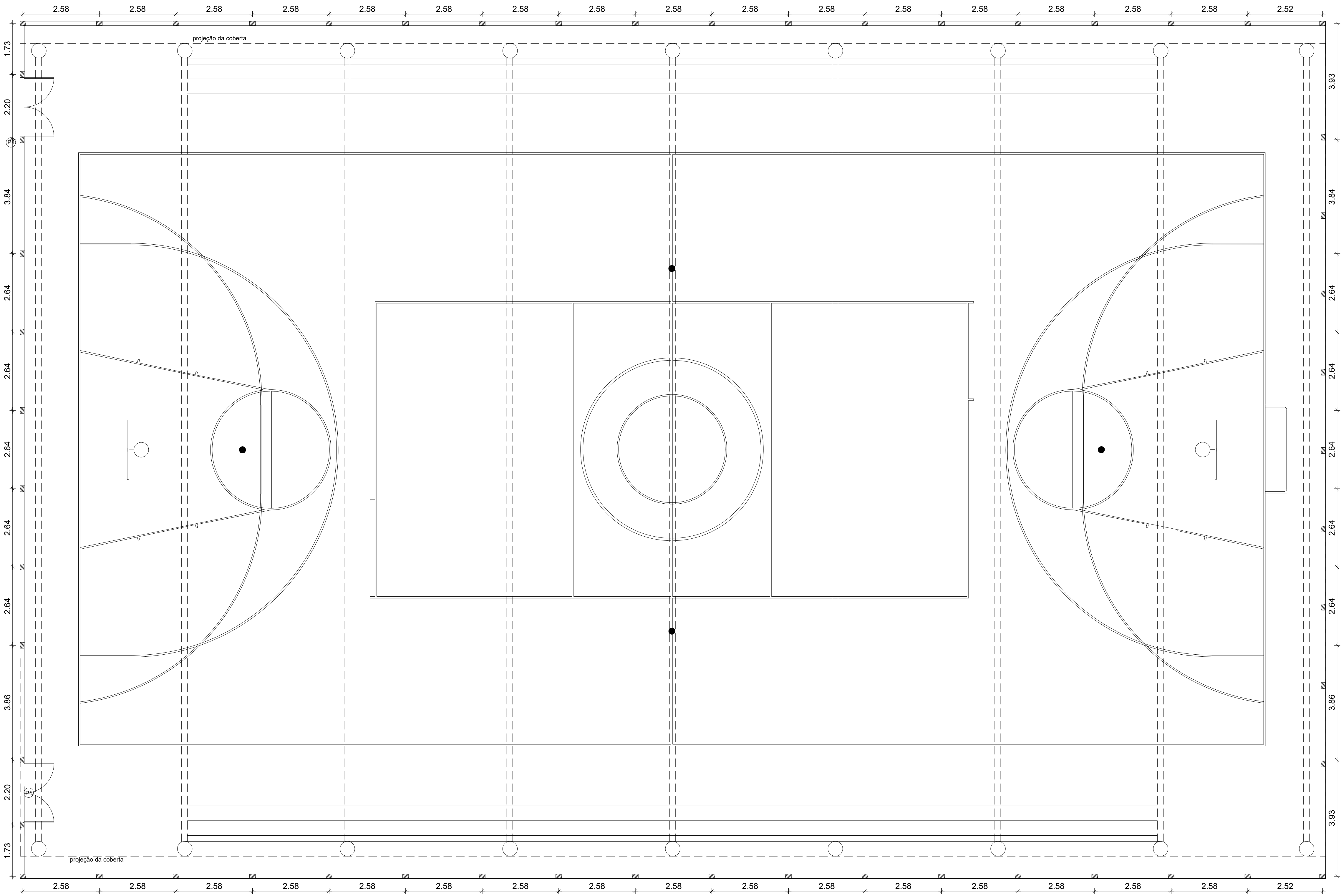
PLANTA BAIXA 1/75
