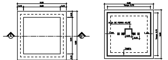
PLANTA BAIXA
