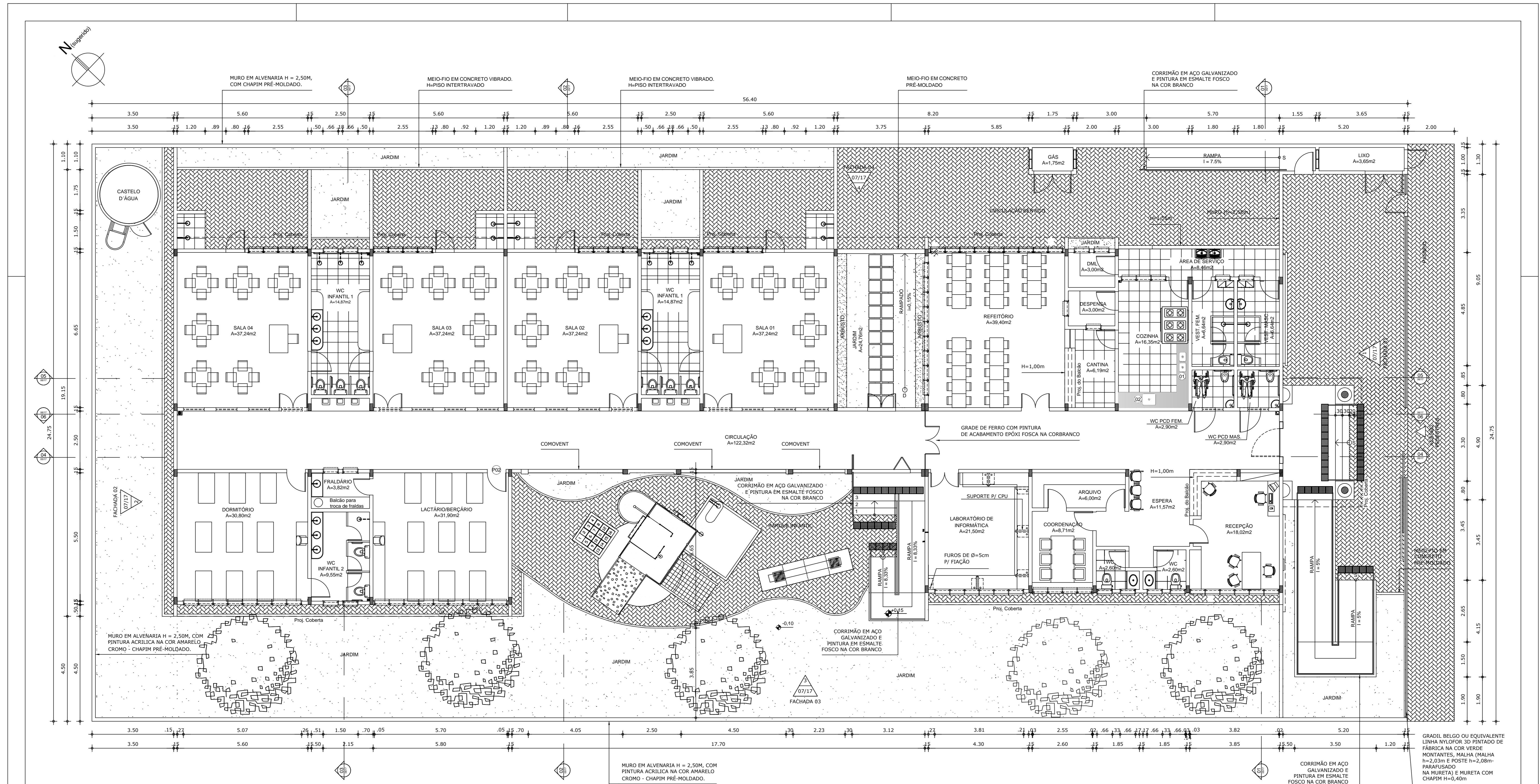
01 PLANTA DE LAYOUT ESCALA 1/10
