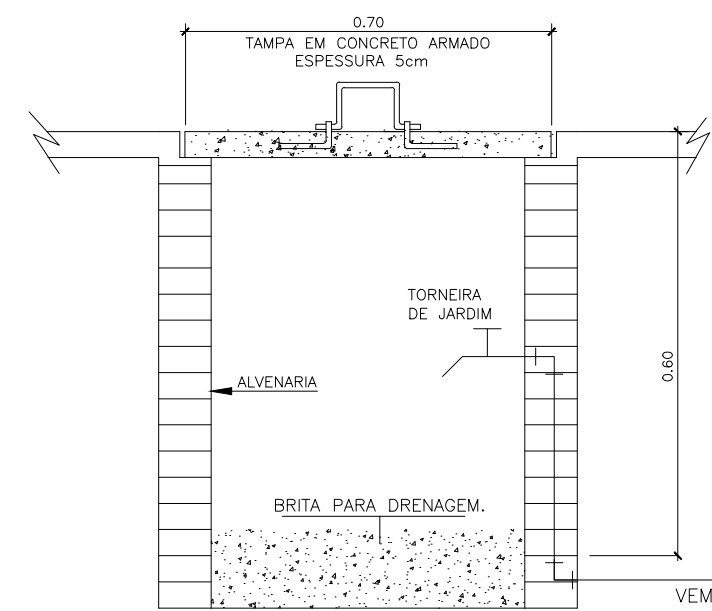
CORTE - A B'
