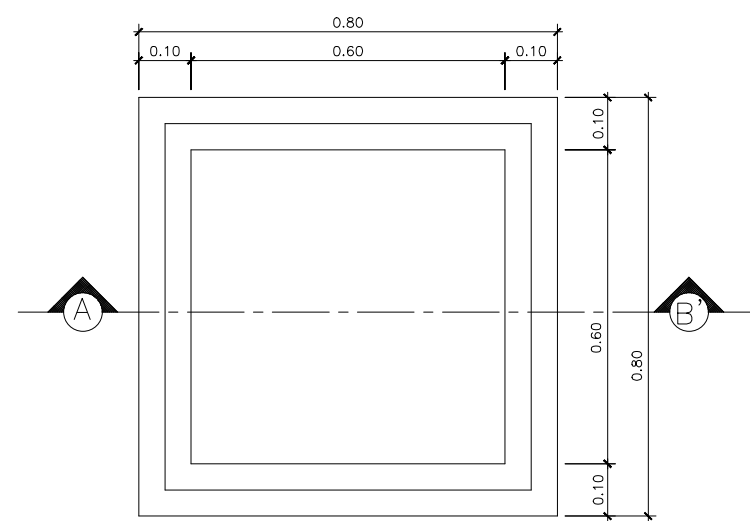
PLANTA BAIXA
