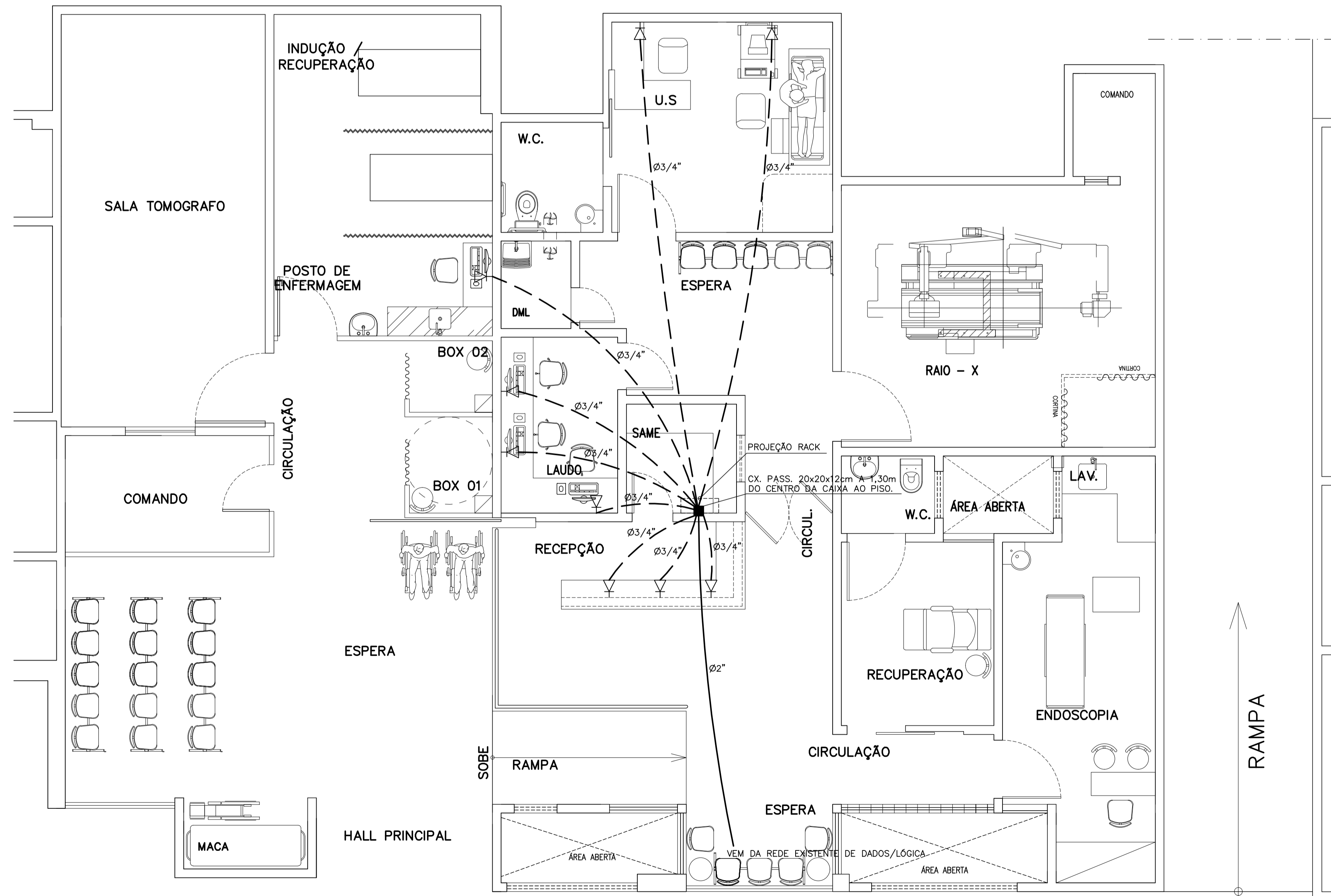
PLANTA BAIXA – CENTRO DE IMAGEM ESCALA 1/50
